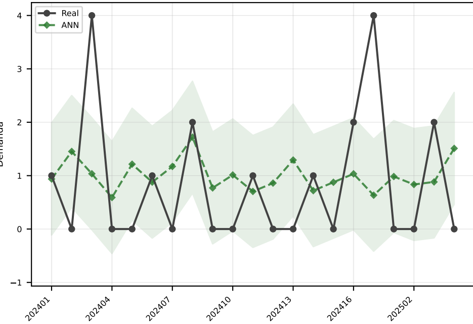
ANN MAE=1.0
