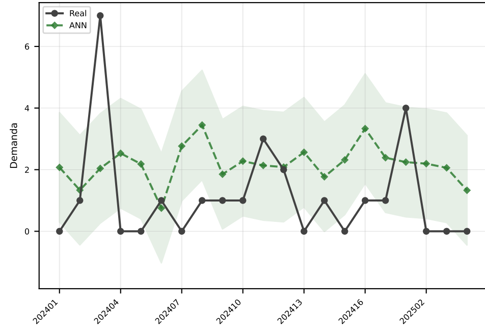
ANN MAE=1.8
