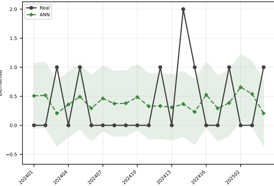
ANN MAE=0.6
