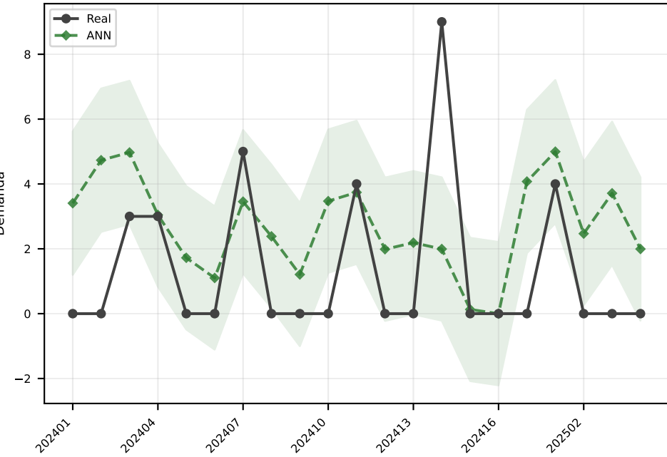
ANN MAE=2.2
