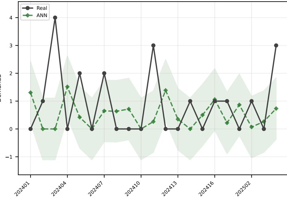
ANN MAE=1.1
