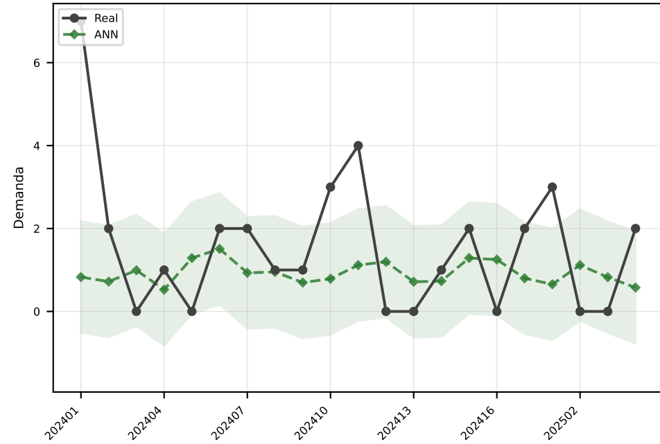
ANN MAE=1.3
