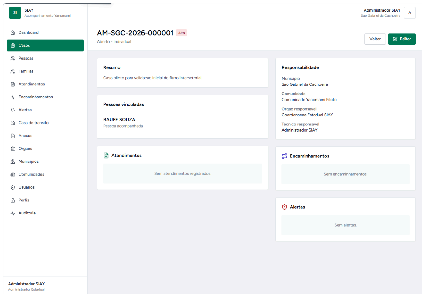
Imagem 4 - Detalhe do caso e historico operacional.
