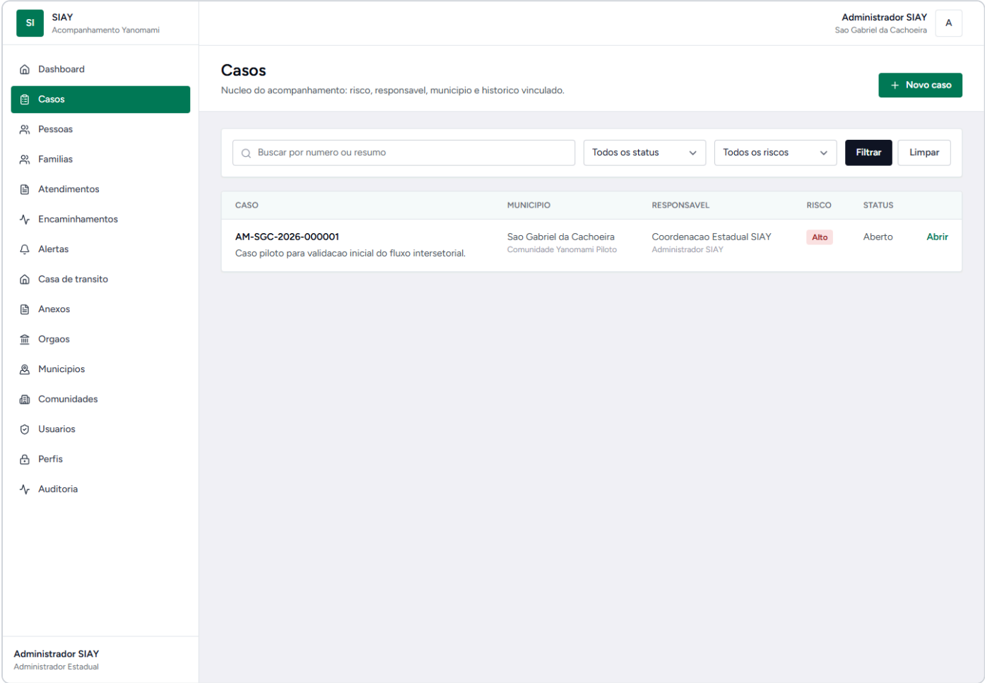
Imagem 3 - Listagem de casos com filtros.
