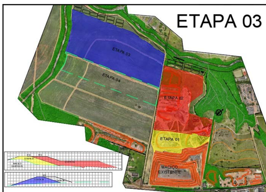
Figura 17: Representação esquemática da Etapa 3 de ampliação
