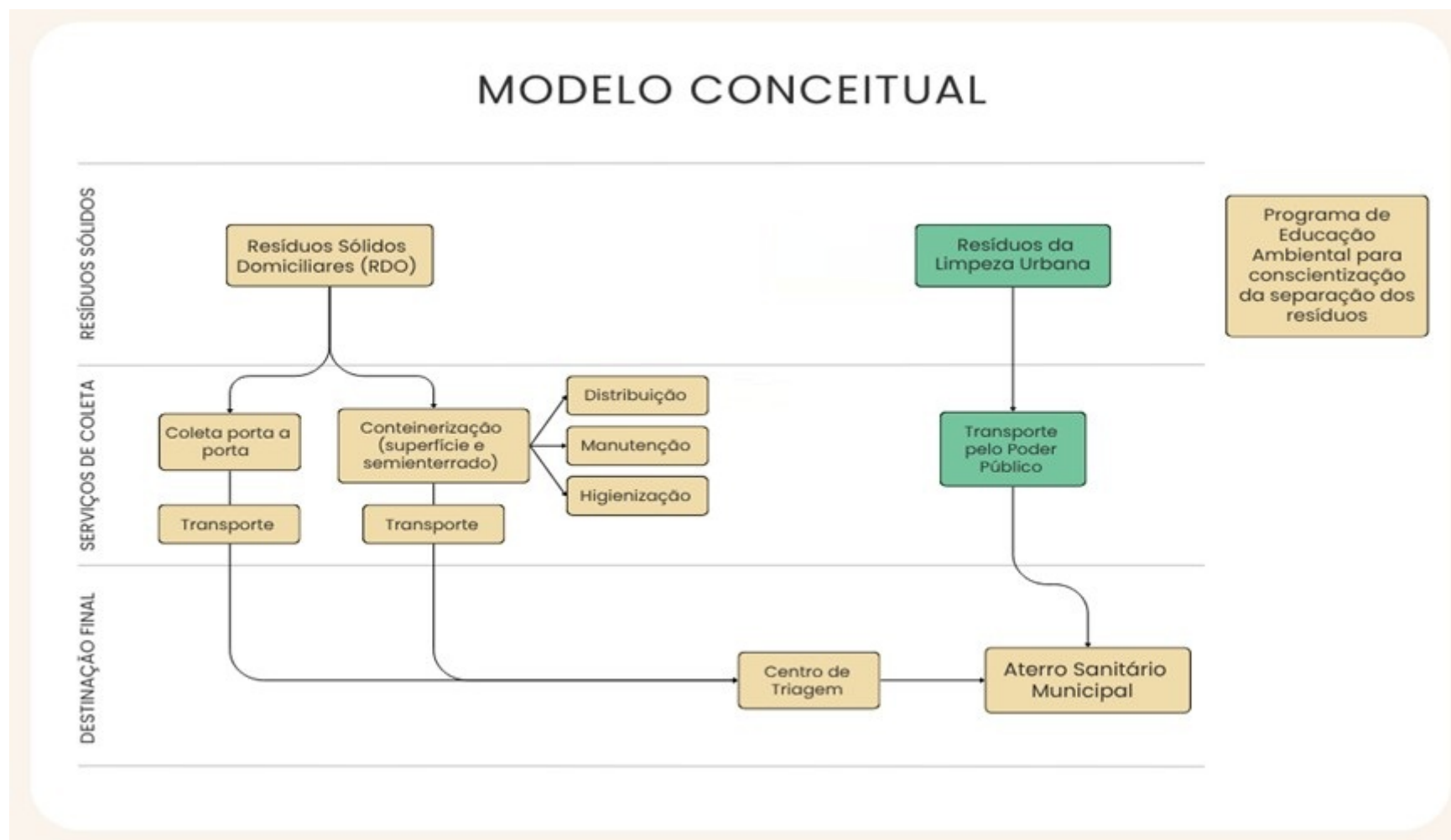
Figura 8 – Modelo Conceitual do Sistema Integrado de Manejo de Resíduos Sólidos
