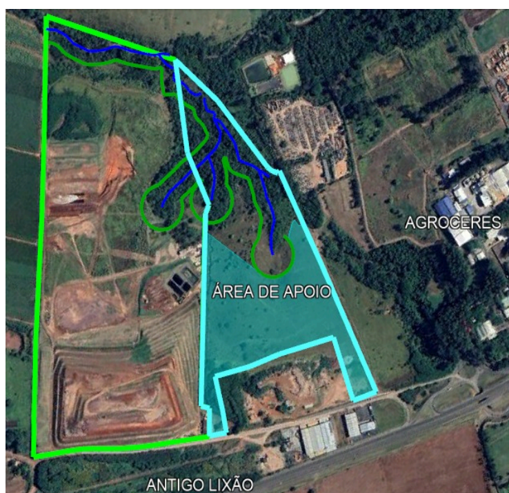
Figura 19: Área prevista para implantação das novas estruturas operacionais
