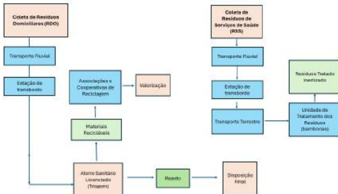
FIGURA 1 – ROTA TECNOLÓGICA REFERENCIAL PARA O BAIXO MADEIRA
