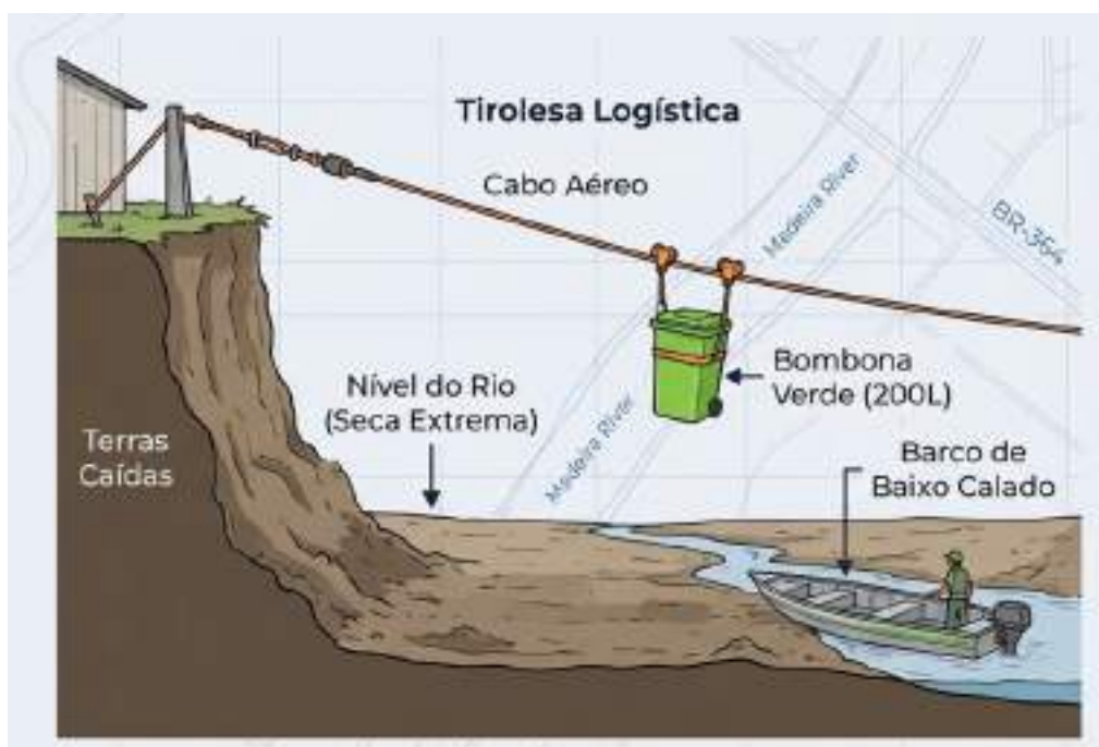
FIGURA 6 – SOLUÇÃO REFERENCIAL DE TRANSPOSIÇÃO/APOIO EM CENÁRIO DE ESTIAGEM
