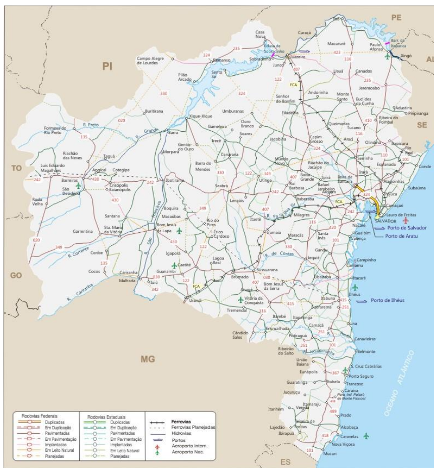
Figura 01 - Mapa Rodoviário da Região do CDS VELHO CHICO Fonte: Secretaria de Infraestrutura do estado da Bahia, 2023
