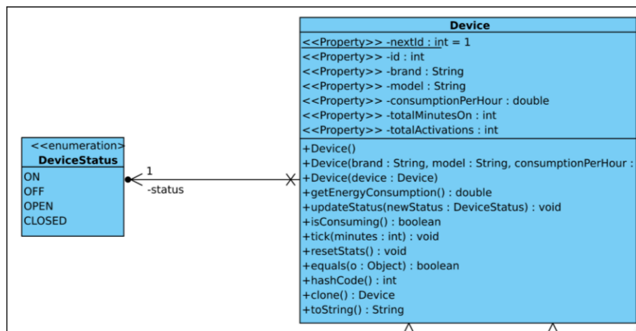
Figura 1: Diagrama de classes da classe Device
