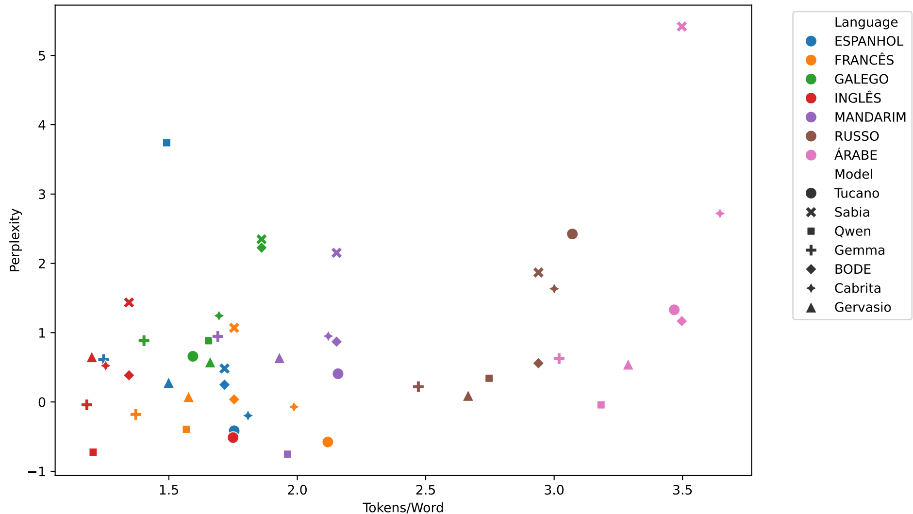
causalLM - RELATAR
