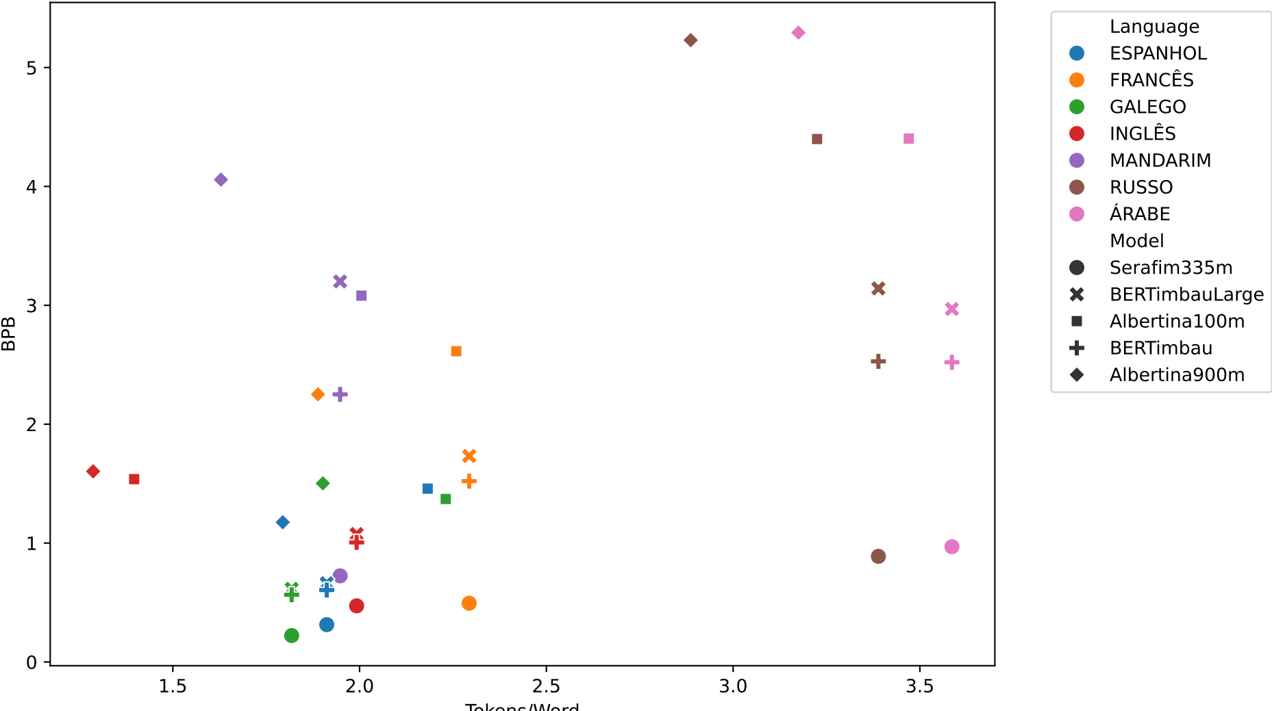
maskedLM - EXPLORAR
