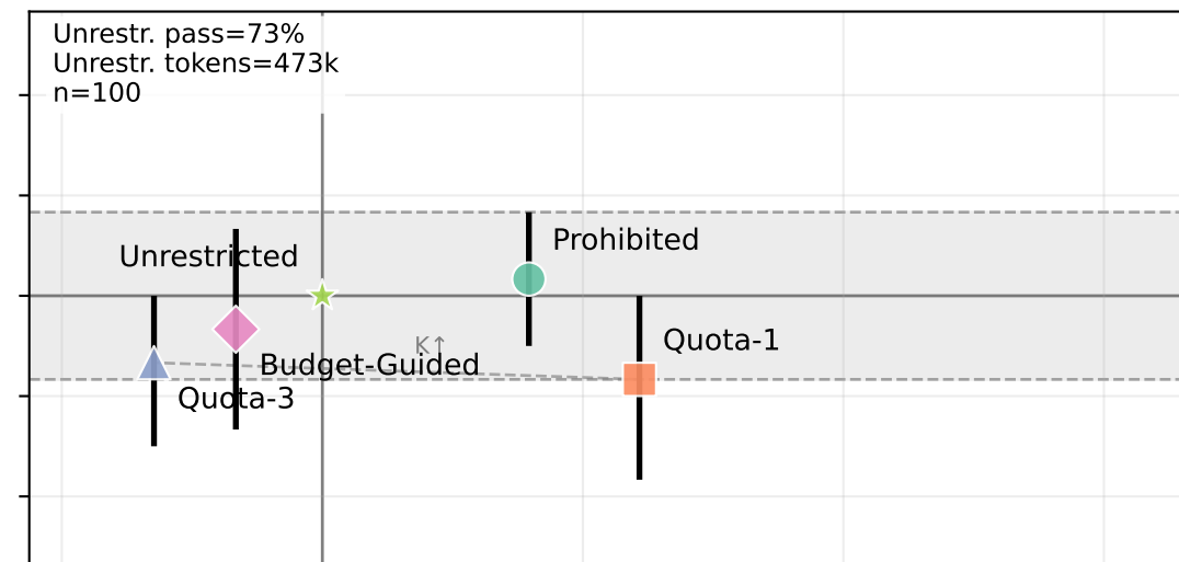
SWE-bench Lite — Codex
