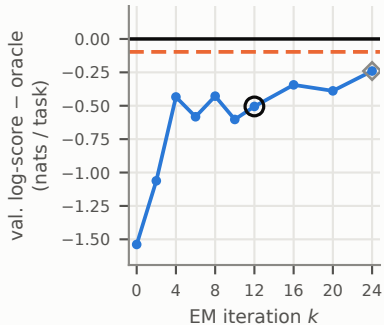
IW, RI ( d = 8 )
