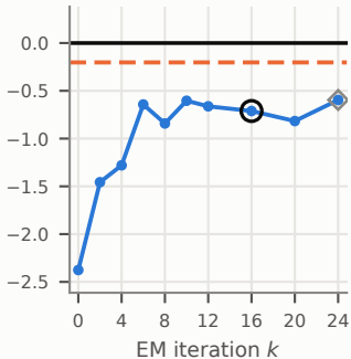
IW, non-RI ( d = 8 )
