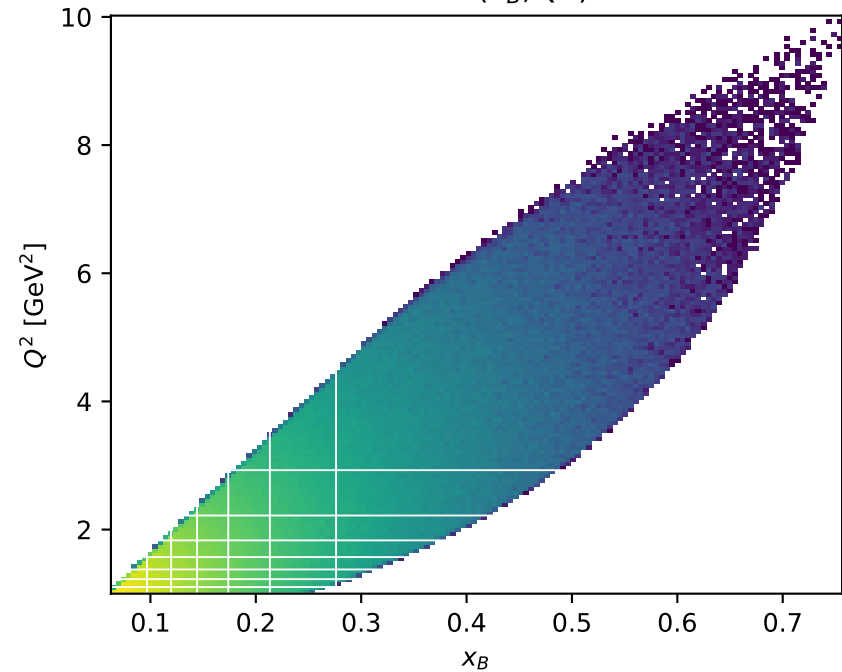
Grid A ( x_B, Q^2 )
