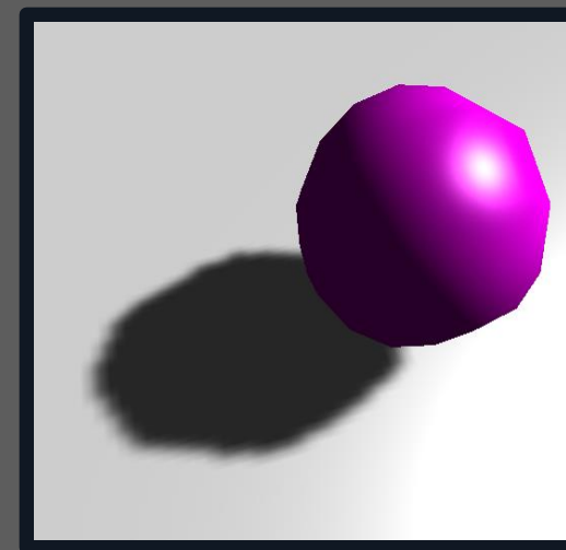
PCF(3x3)
