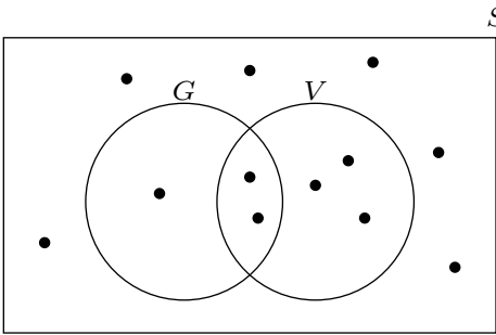
Venn diagram
