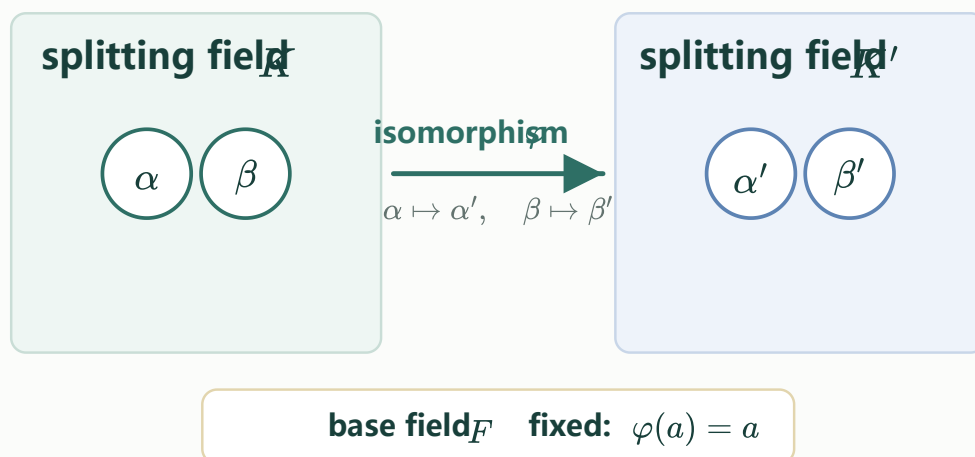
图 4: 两个 splitting field 可以不是同一个集合, 但有一个固定 base field 的结构保持对应。
