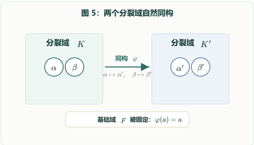
两个分裂域自然同构
