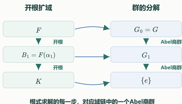
图 8：根式求解与可解群的平行流程
