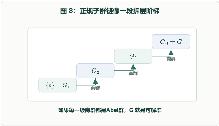
正规子群链阶梯图
