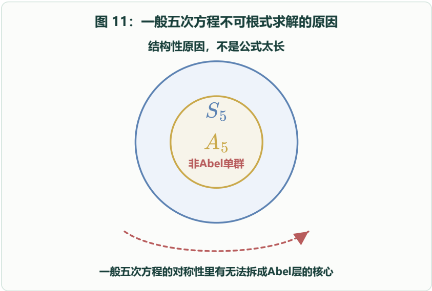
图 11：S5 中的 A5 是一般五次方程不能用根式通解的结构原因
