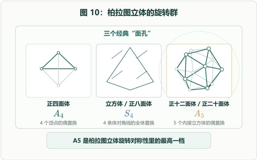
图 10：柏拉图立体的旋转群
