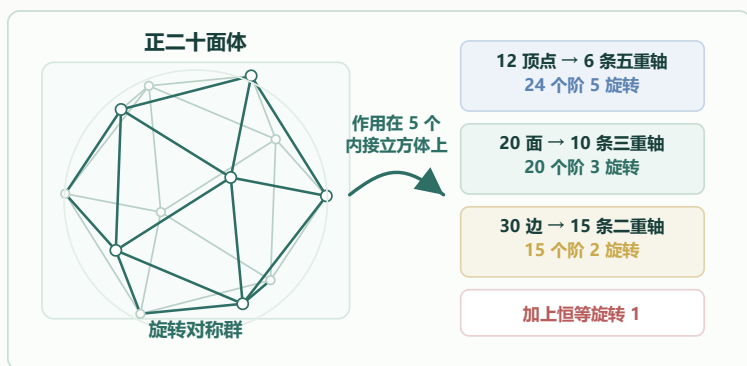
图 9: A_5 与正二十面体旋转对称
