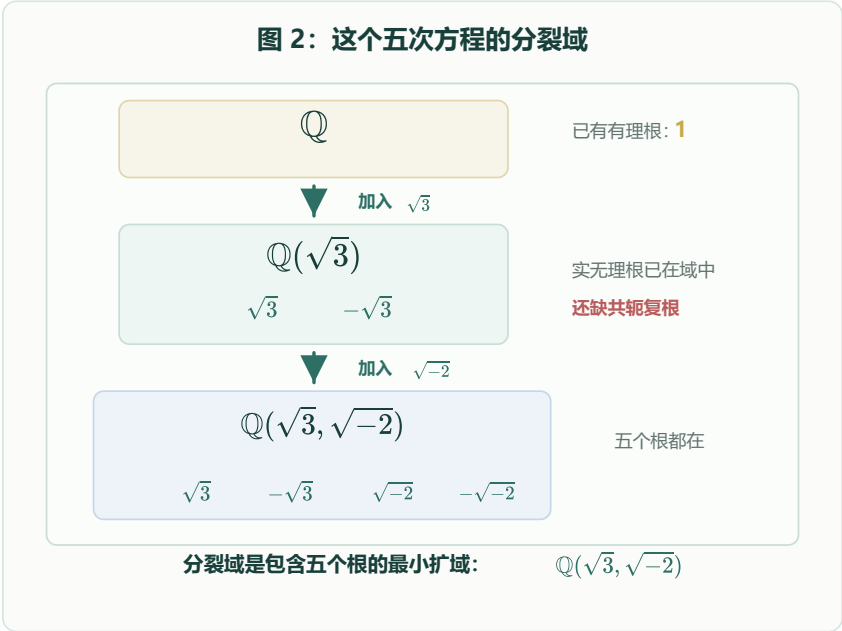
图 2：为了让这个五次多项式完全分裂，需要把实无理根和共轭复根都加入基础域。
