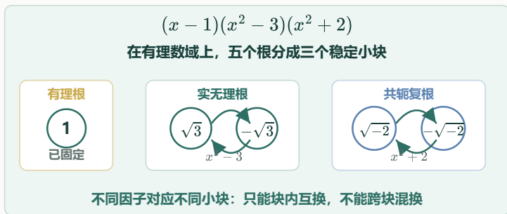
图 1：一个五次方程里的三类根
