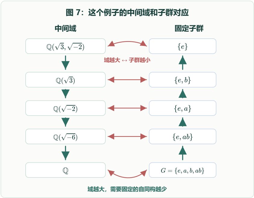
Galois 基本定理的域链和群链对应
