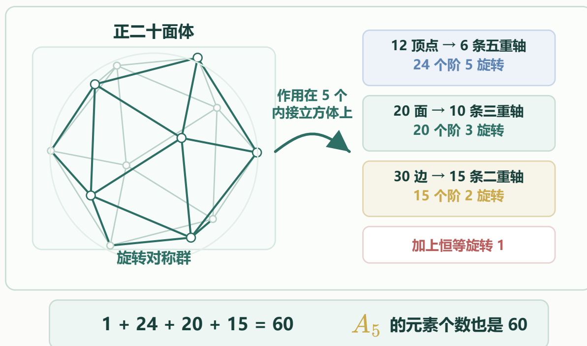
图 9: A_5 与正二十面体旋转对称
