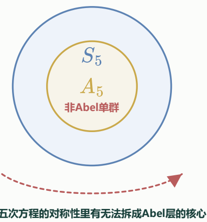
图 11：一般五次方程不可根式求解的原因 结构性原因，不是公式太长
