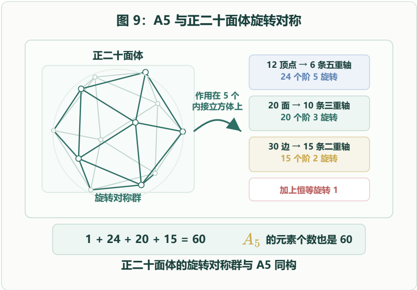
A_5 与正二十面体旋转对称群
