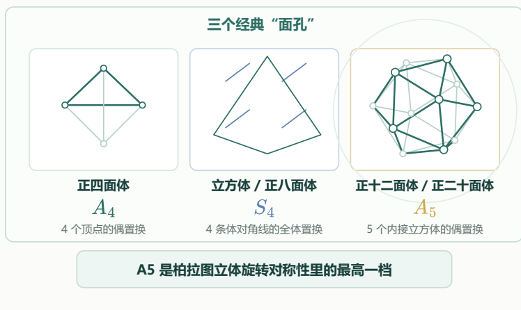
图 10：柏拉图立体的旋转群
