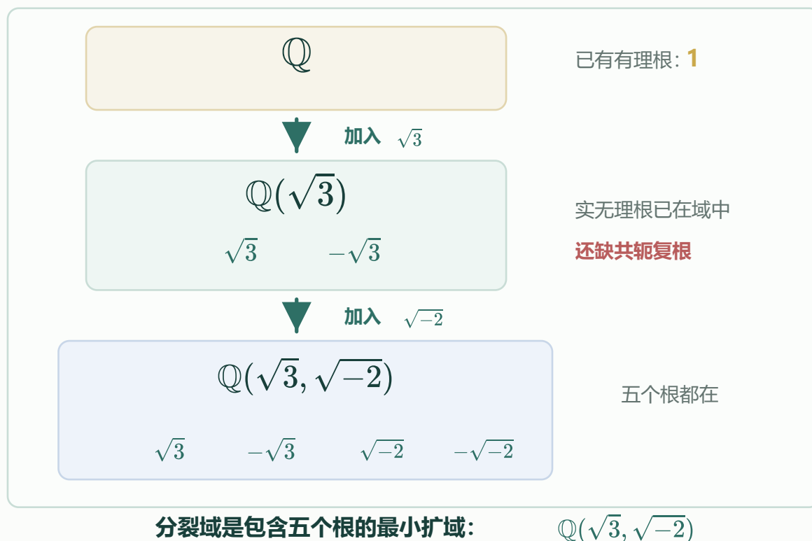
图 2: 这个五次方程的分裂域
