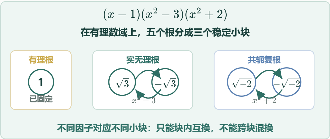
图 1：一个五次方程里的三类根
