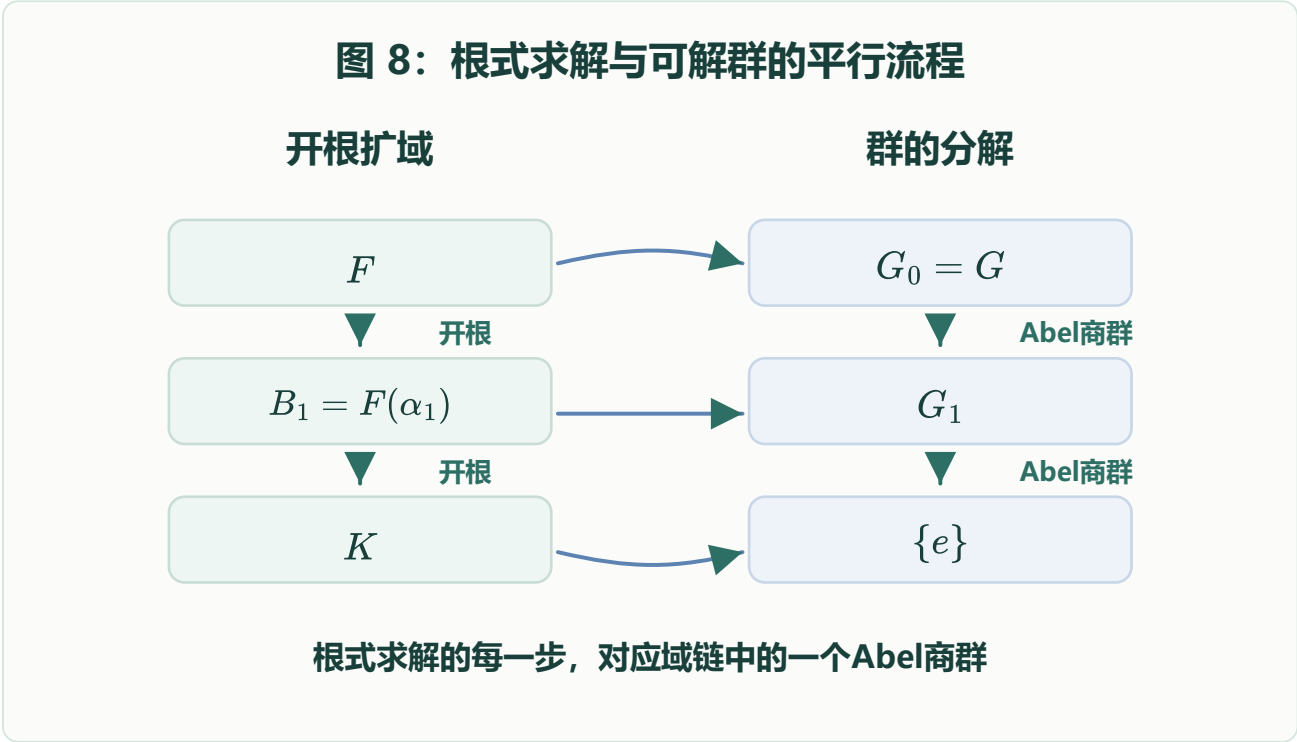
图 8：根式求解给出一串域扩张；Galois 理论把这串域扩张翻译成一串正规子群和 Abel 商群。
