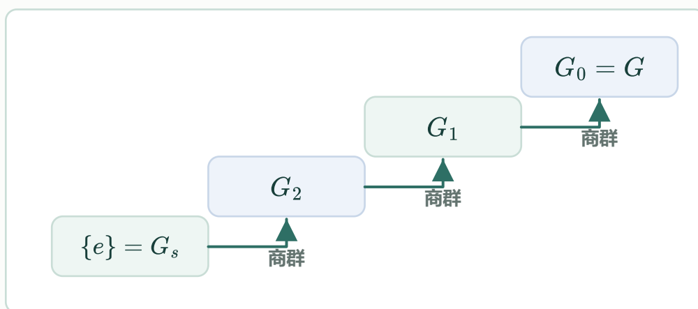
图 8：正规子群链像一段拆层阶梯
