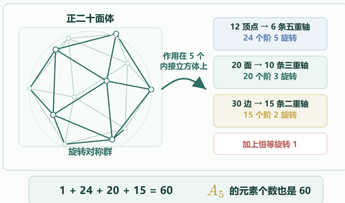
图 9: A_5 与正二十面体旋转对称
