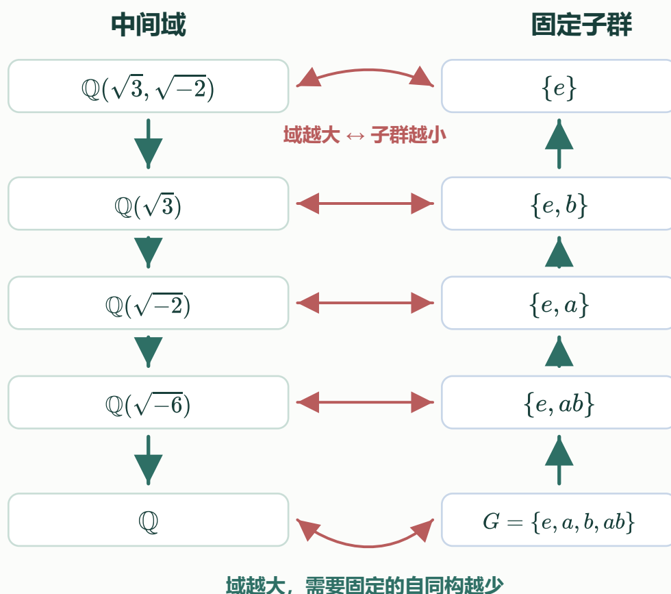
图 7：这个例子的中间域和子群对应
