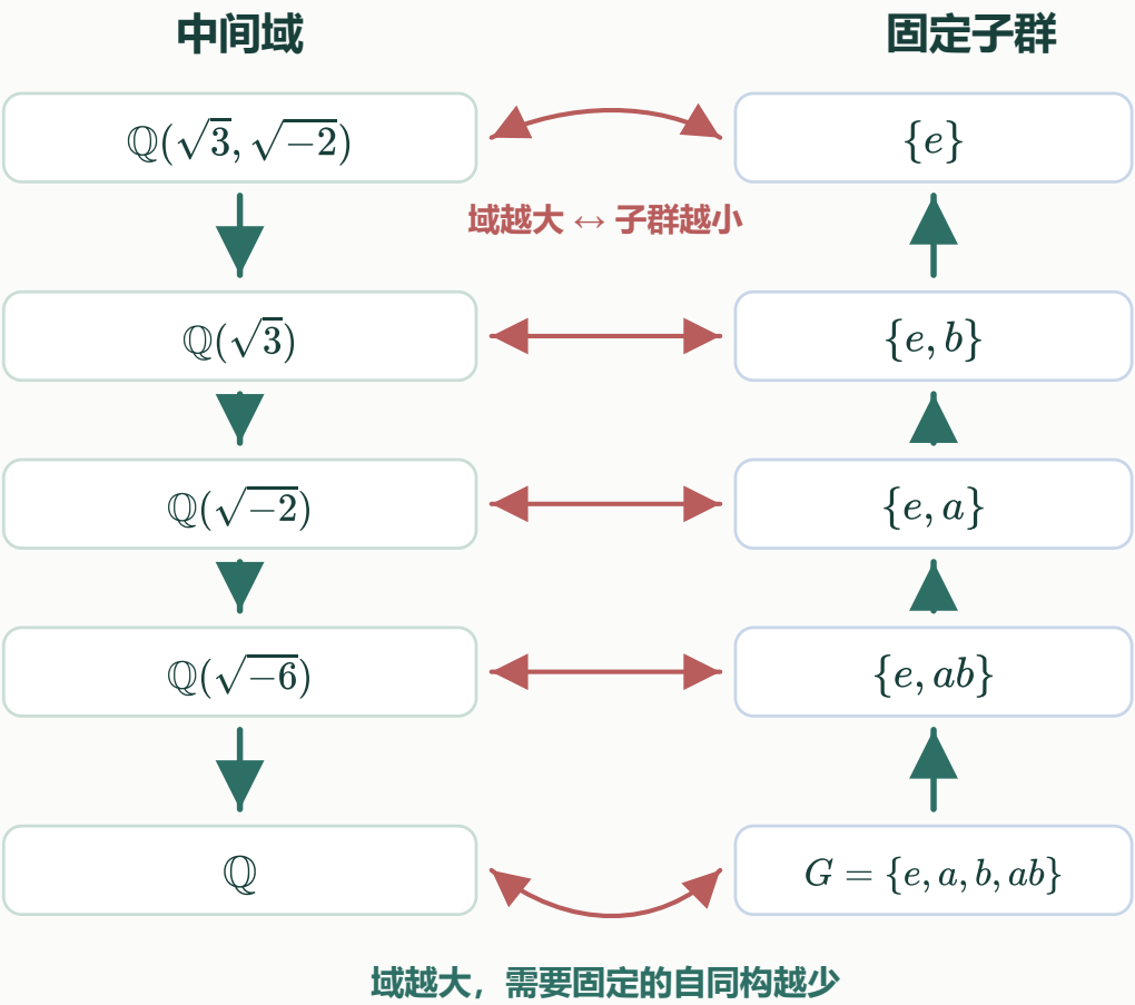
图 7：这个例子的中间域和子群对应
