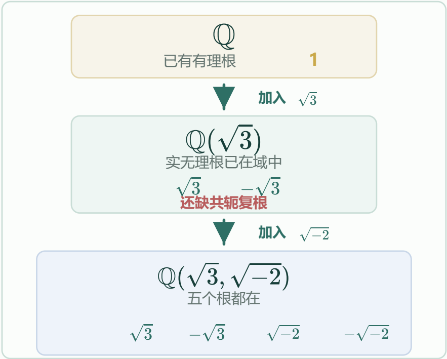
图 2：这个五次方程的分裂域
