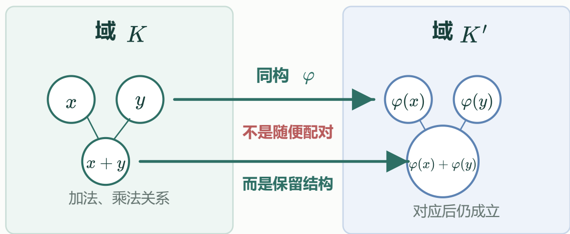
图 5a：同构是保留加法和乘法结构的一一对应
