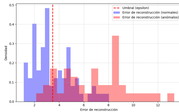
Figura 3.3: Distribución del error de reconstrucción para el autocodificador B.
