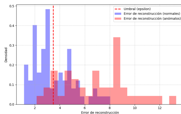
Figura 3.4: Distribución del error de reconstrucción para el autocodificador C.
