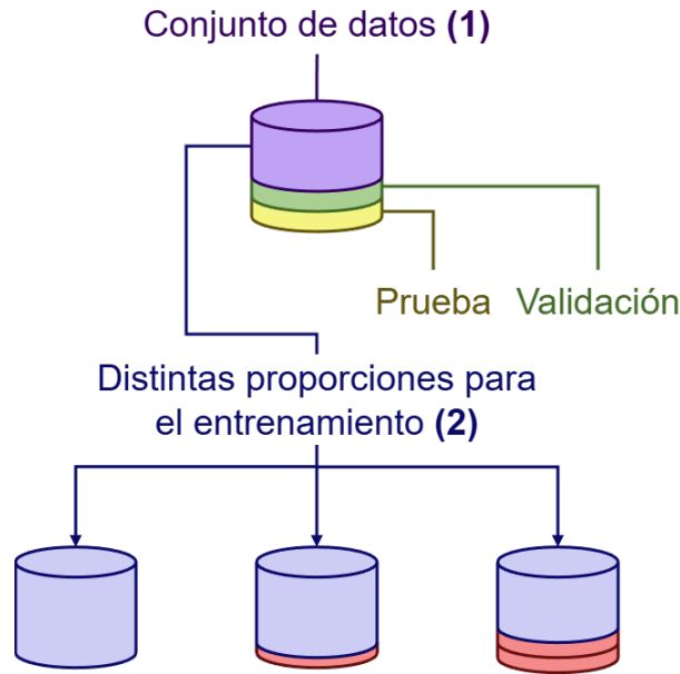
Figura 2.3: Diagrama del proceso de división del conjunto de datos en entrenamiento, validación y prueba, para posterior creación de los subconjuntos A, B y C con diferentes proporciones de anomalías.
