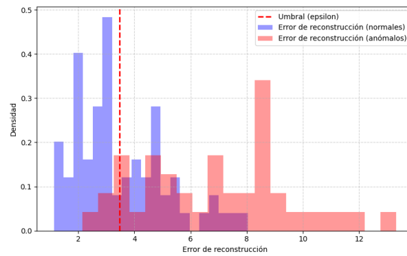
Figura 3.2: Distribución del error de reconstrucción para el autocodificador A.
