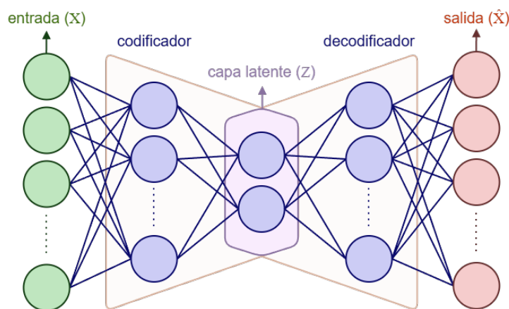
Figura 2.4: Arquitectura de un autocodificador: la entrada X es procesada por el codificador hasta obtener la representación latente Z , a partir de la cual el decodificador reconstruye la salida \hat{X} .
