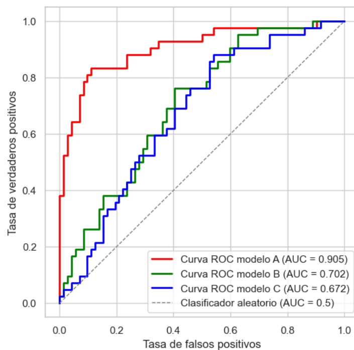
Figura 3.8: Curvas ROC y AUC obtenidos para los modelos AE, SAE y CAE entrenados con el Conjunto A (0 % de anomalías).
