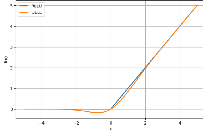
Figura 2.5: Comparación entre las funciones de activación ReLU y GELU. Se observa que GELU presenta una transición suave alrededor de cero, lo que evita discontinuidades y favorece un entrenamiento más estable en modelos neuronales.
