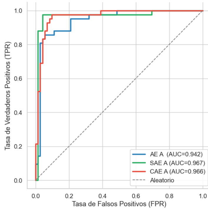
Figura 3.7: Curvas ROC y AUC obtenidos para los modelos AE, SAE y CAE entrenados con el Conjunto A (0 % de anomalías).
