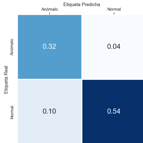
Figura 3.4: Matriz de confusión para el modelo A expresada en valores relativos.
