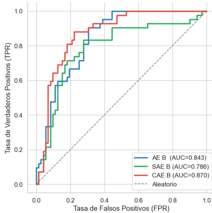
Figura 3.8: Curvas ROC y AUC obtenidos para los modelos AE, SAE y CAE entrenados con el Conjunto B (10 % de anomalías).
