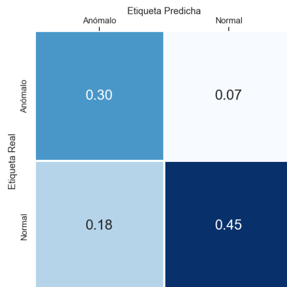
Figura 3.5: Matriz de confusión para el modelo B expresada en valores relativos.
