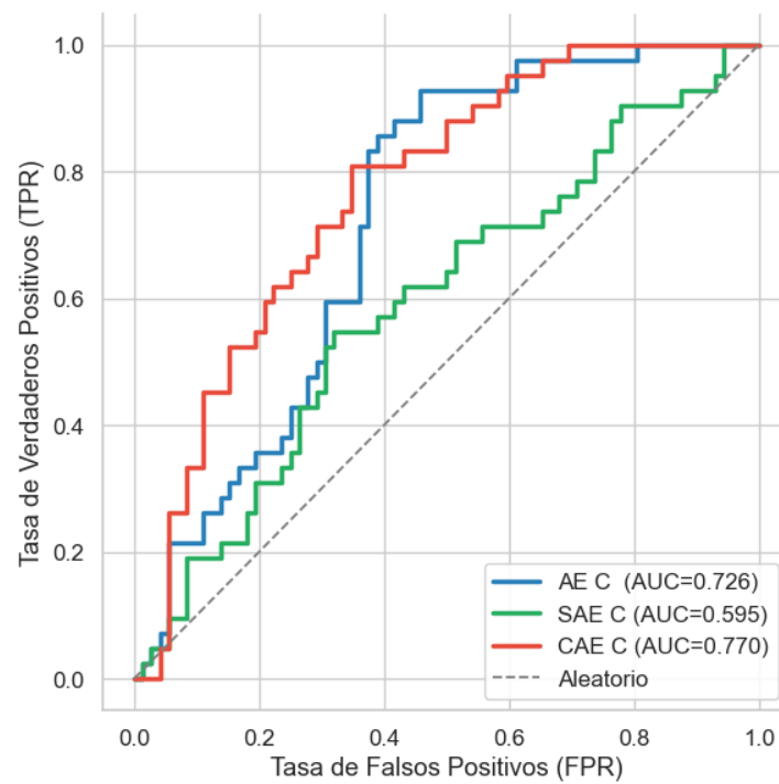
Figura 3.9: Curvas ROC y AUC obtenidos para los modelos AE, SAE y CAE entrenados con el Conjunto C (25 % de anomalías).
