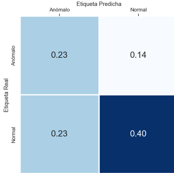
Figura 3.6: Matriz de confusión para el modelo C expresada en valores relativos.
