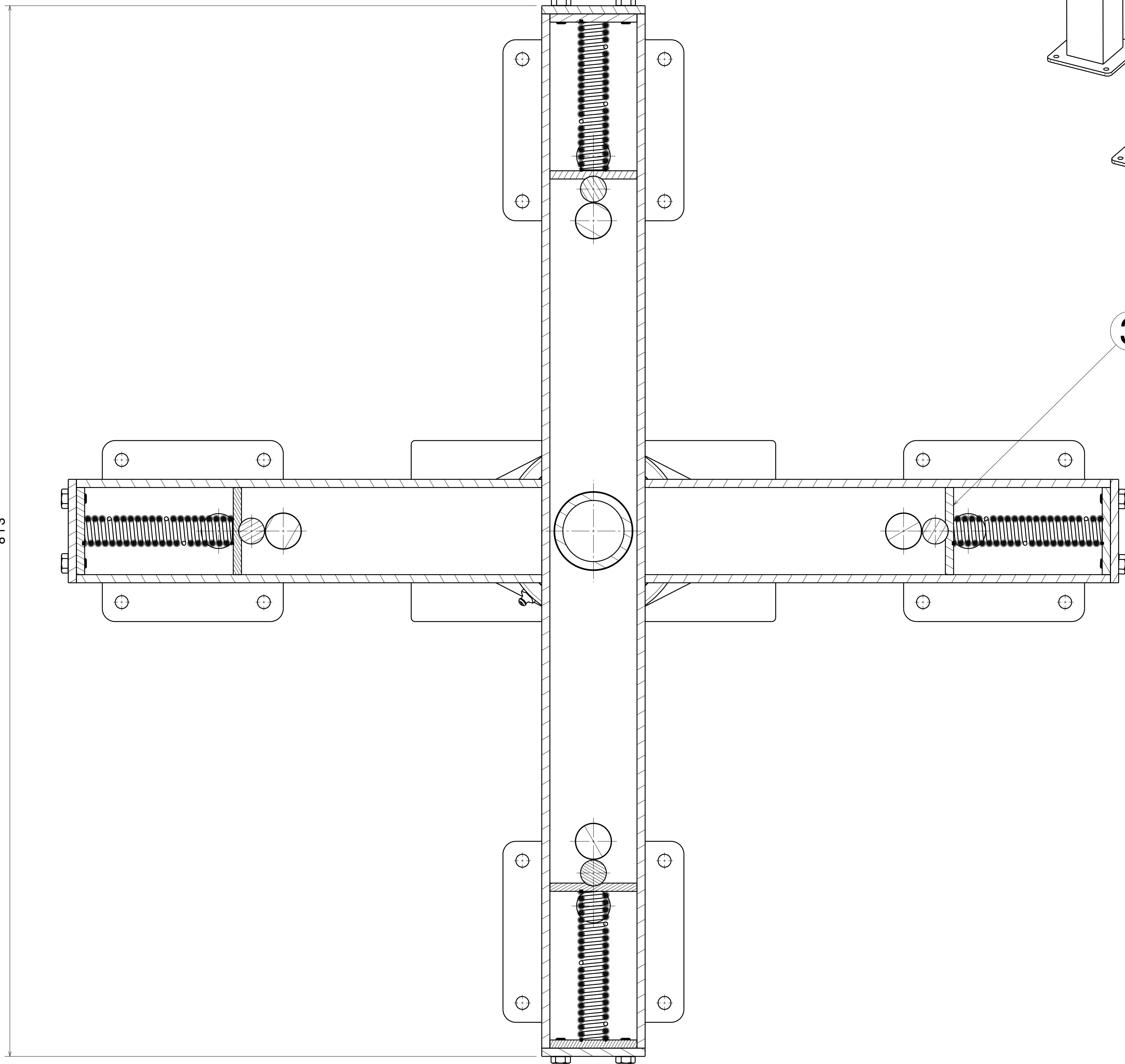
CORTE A-A
