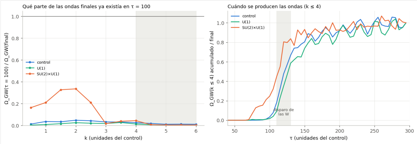
Izquierda: qué parte de las ondas finales ya existía en \tau = 100 , por k. Derecha: ondas acumuladas ( k \leq 4 ) contra el tiempo; la franja gris es el disparo de las W. Hecha con code/produccion_gws.py .
