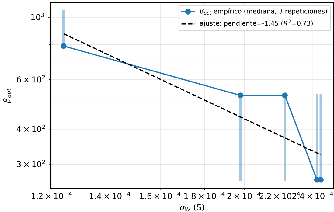
Barrido C: ventana de conductancia (vía \sigma_W )
