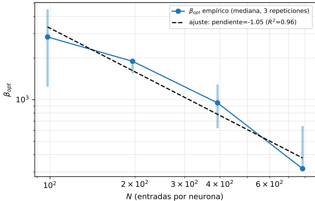
Barrido A: tamaño de la crossbar (SP, MNIST)
