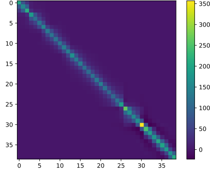
Slika 3: Pasovna struktura Hessove matrike H za n = 40 segmentov trajektorije.
