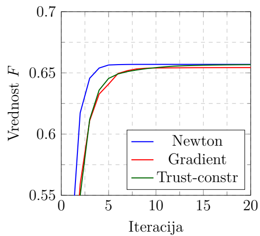
(b) n = 10 točk
