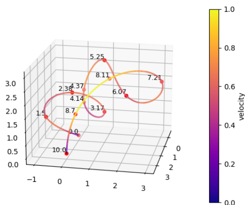
Slika 1: Primer optimalne trajektorije glede na trzaj (3. odvod) in s končnim časom 10 s, kjer so z rdečimi pikami podane vmesne točke, ob njih pa so pripisani pripadajoči vmesni časi.
