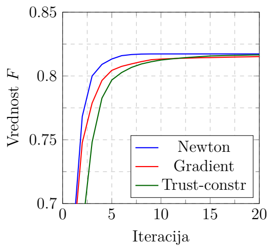
(b) n = 10 točk
