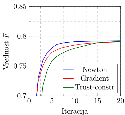
(d) n = 30 točk
