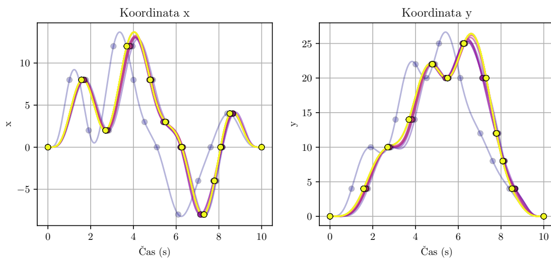
Slika 4: Analiza konvergence za n = segmentov trajektorije.
