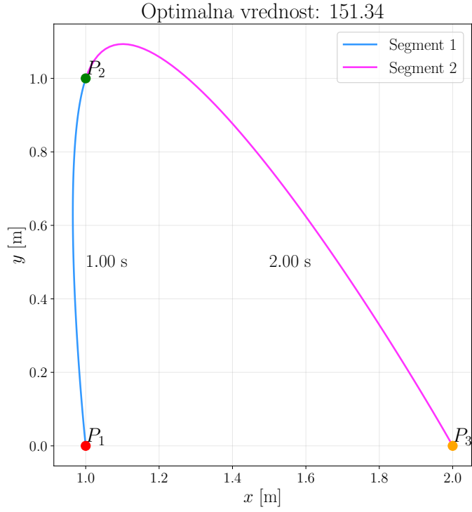
Slika 7: Trajektorija, dobljena z rešitvijo QP problema za n = 2 segmenta, d = 4 , K = 2 in r = 3 .
