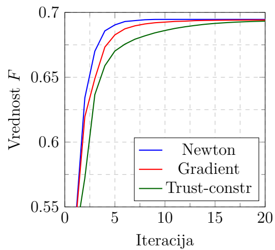
(d) n = 30 točk
