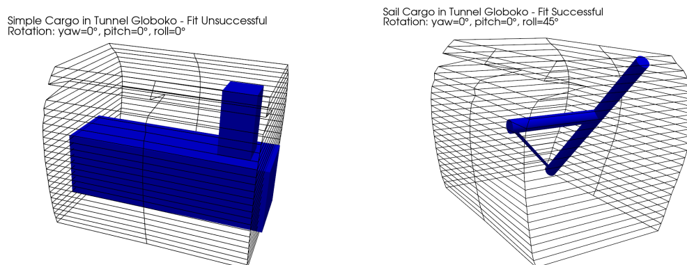
Slika 6.5: Prileganje tovora v prilagojeni model vagona za predor Globoko: neuspešno prileganje enostavne zaboje (levo) in uspešno prileganje tovora v obliki jadra (desno).
