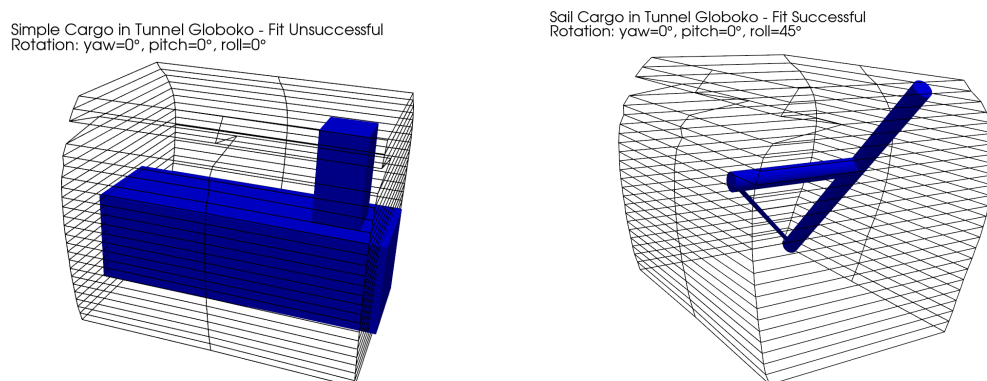
Slika 6.5: Prileganje tovora v prilagojen model vagona za predor Globoko: neuspešno prileganje enostavne zaboje (levo) in uspešno prileganje tovora v obliki jadra (desno).
