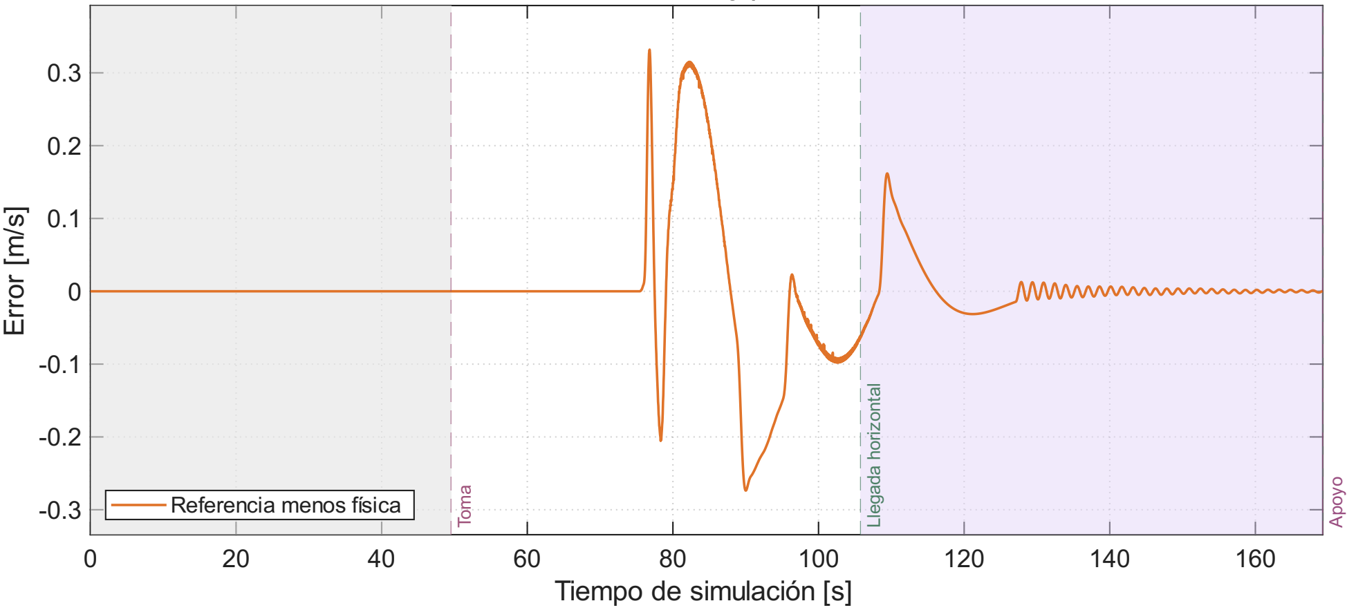
CODESYS automático con antisway | Error de velocidad del carro
