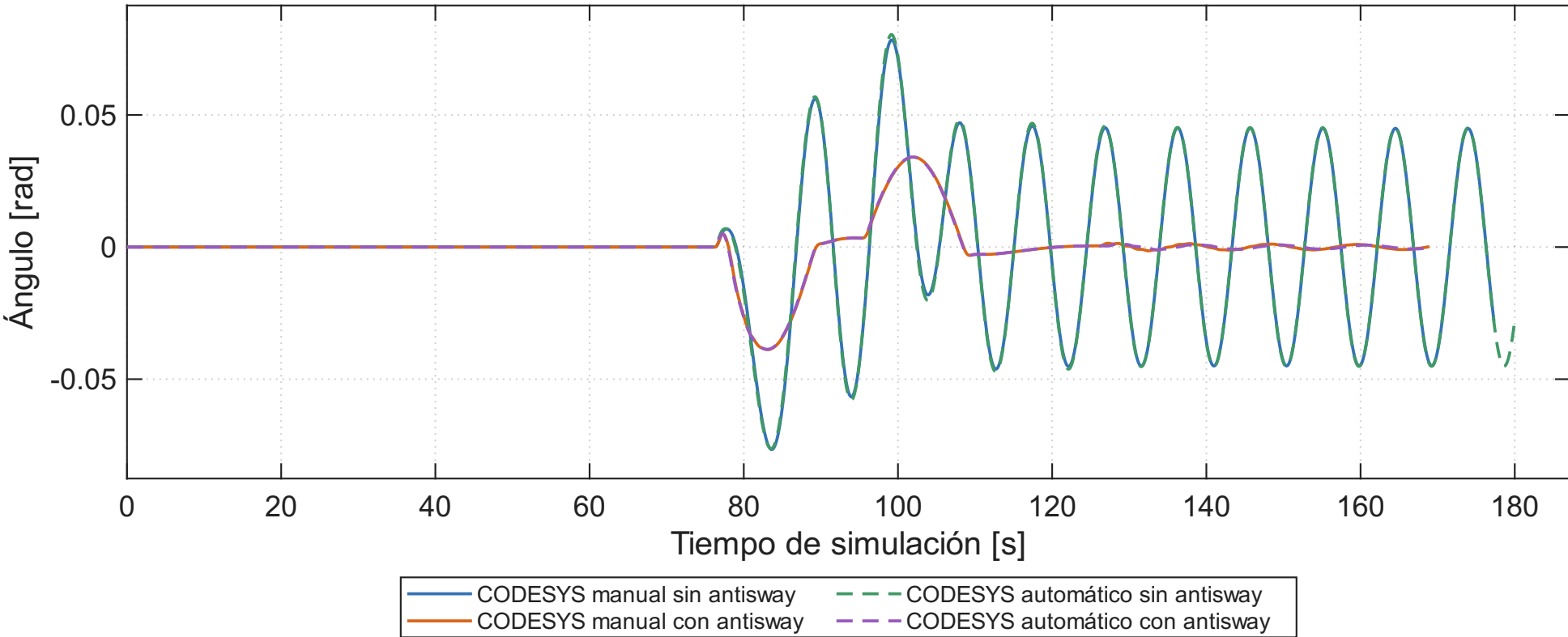
Comparación de las cuatro pruebas | Ángulo del péndulo
