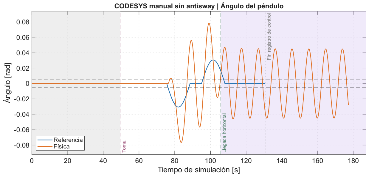
Figura 86: CODESYS manual sin antisway: Ángulo físico y de referencia del péndulo. Las líneas horizontales señalan los umbrales angulares del descenso. Se respeta la cobertura parcial de las señales y no se extrapolan datos faltantes.
