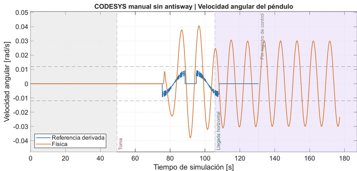
Figura 87: CODESYS manual sin antisway: Velocidad angular física y referencia derivada numéricamente; se distinguen ambas fuentes. Las líneas horizontales indican los umbrales del descenso. Se respeta la cobertura parcial de las señales y no se extrapolan datos faltantes.
