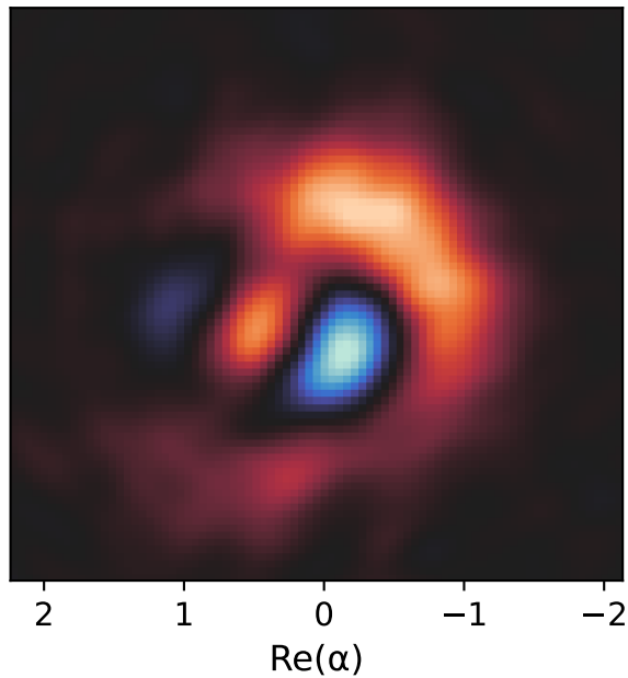
QST-CGAN
