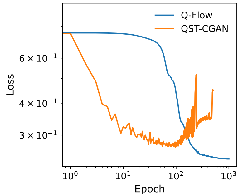
QST-CGAN
