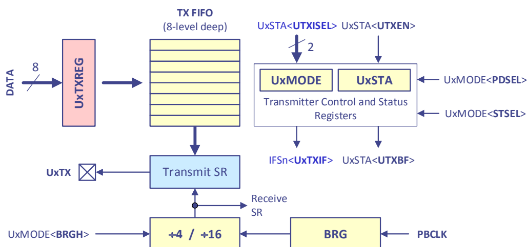
Figura 1. Diagrama de blocos simplificado do módulo de transmissão da UART.
