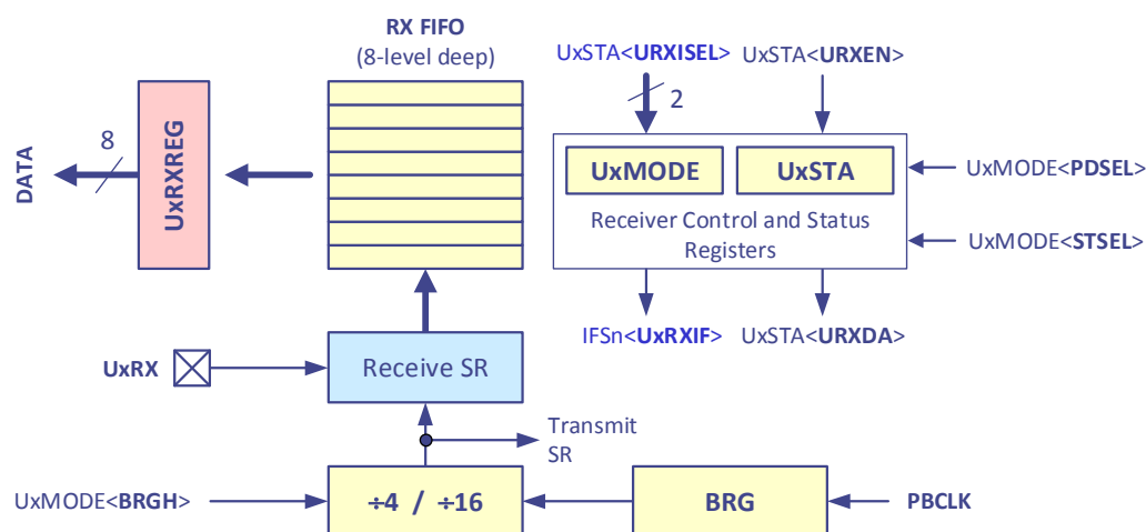
Figura 2. Diagrama de blocos simplificado do módulo de receção da UART.
