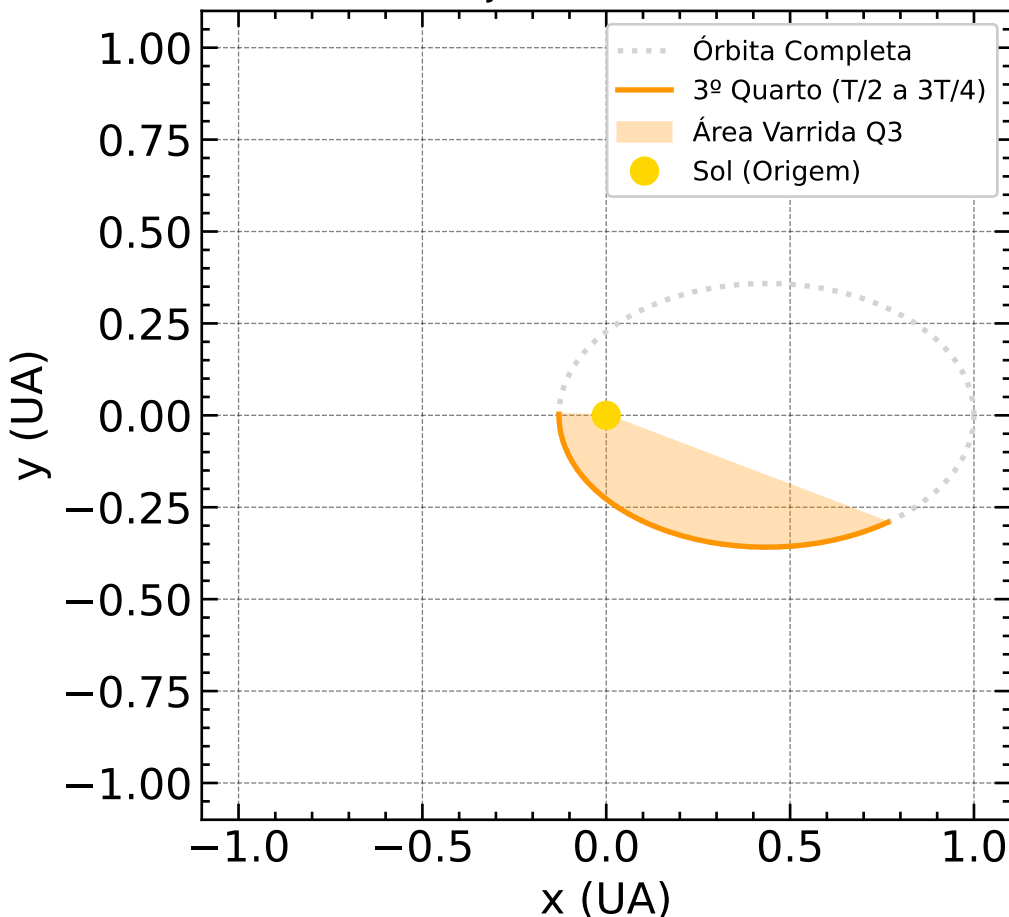
Quarto 3 da Trajetória (Área: 0.158850 UA 2 )
