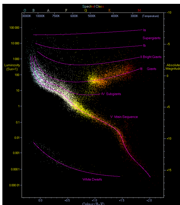
Figura 3 – O diagrama Hertzsprung-Russell para 22.000 estrelas do Catálogo Hipparcos e 1.000 anãs vermelhas e brancas do Catálogo Gliese, destacando a Sequência Principal, onde estrelas como o Sol se situam entre o canto superior esquerdo e o inferior direito.
