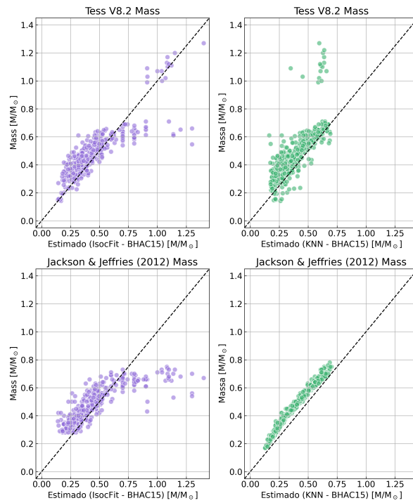
Figura 20 – Gráficos comparativos das estimativas de massa para NGC 2516, similar aos gráficos da Figura 18, mas aplicados ao aglomerado NGC 2516.
