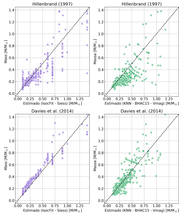
Figura 12 – Comparação entre as estimativas de massa utilizando diferentes métodos de ajuste de isócronas e magnitudes para dois conjuntos de dados distintos: Hillenbrand (1997) e Davies et al. (2014). Cada linha de gráficos corresponde a um conjunto de dados, e cada coluna refere-se a uma metodologia de estimativa.
