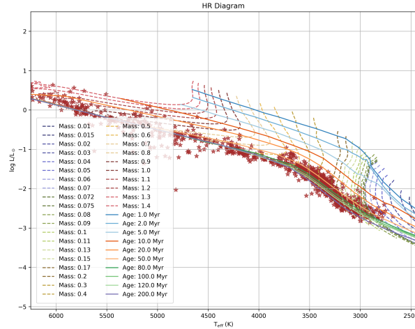
Figura 17 – Diagrama HR que mostra a relação entre luminosidade e temperatura das estrelas do aglomerado das Plêiades. As linhas sólidas representam as isócronas teóricas do modelo BHAC15 de Baraffe et al. (2015), enquanto as linhas tracejadas representam trilhas evolutivas com massa constante. As estrelas-alvo das Plêiades estão marcadas com uma estrela vermelha.
