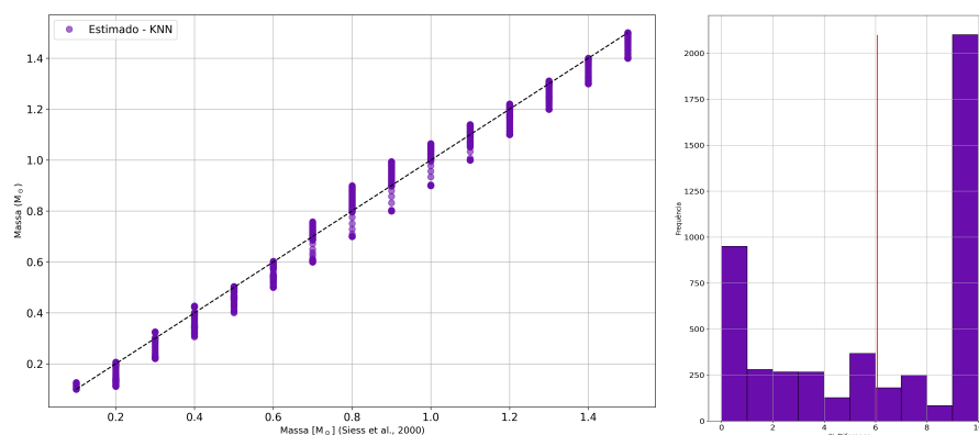
Figura 8 – Análise comparativa e residual do método de ajuste de isócronas para massas de estrelas sintéticas. Esses gráficos comparam as massas estelares estimadas obtidas do método de ajuste de isócronas com as massas obtidas de Siess et al. (2000). A linha sólida, no primeiro, representa a relação ideal de um para um, enquanto os pontos ilustram as previsões, que se alinham estreitamente com os valores observados. O histograma, à direita, representa os resíduos e, apesar de pequenos desvios, o método apresenta boa precisão na estimativa da massa estelar com a mediana demarcada pela linha vermelha.
