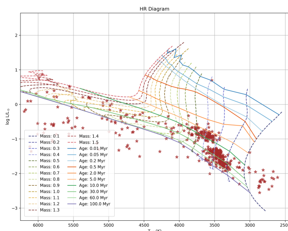
Figura 13 – Mesmo que a Figura 11 para o aglomerado de Upper Scorpius
