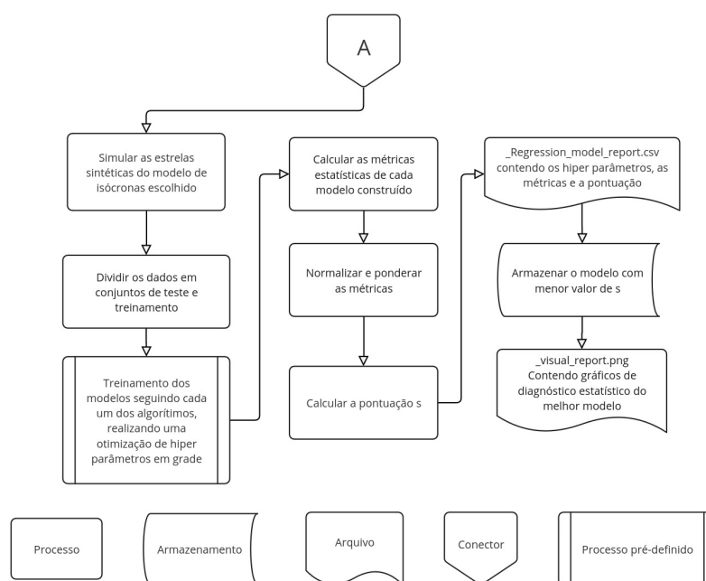
Figura 7 – Fluxograma do processo de treinamento e avaliação de modelos na estimativa de massa estelar.
