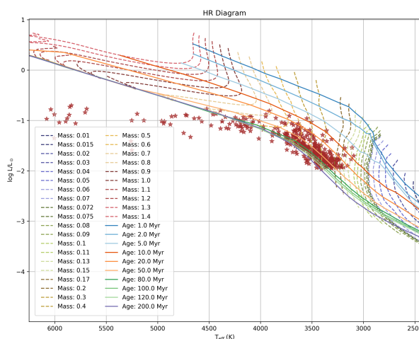
Figura 19 – Diagrama HR para o aglomerado NGC 2516, similar ao gráfico da Figura 17, mas aplicado a NGC 2516.
