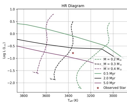
Figura 5 – Determinação de massa utilizando o método de ajuste de isócronas. No gráfico está o DHR para uma estrela do ONC.
