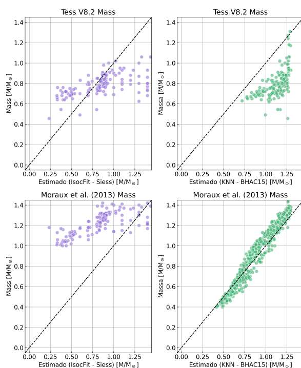
Figura 16 – Comparação entre estimativas de massa utilizando diferentes métodos de ajuste de isócronas e magnitudes para dois conjuntos de dados: TESS V8.2 e Moraux et al. (2013). Cada linha de gráficos refere-se a um conjunto de dados, e cada coluna a um método de estimativa.
