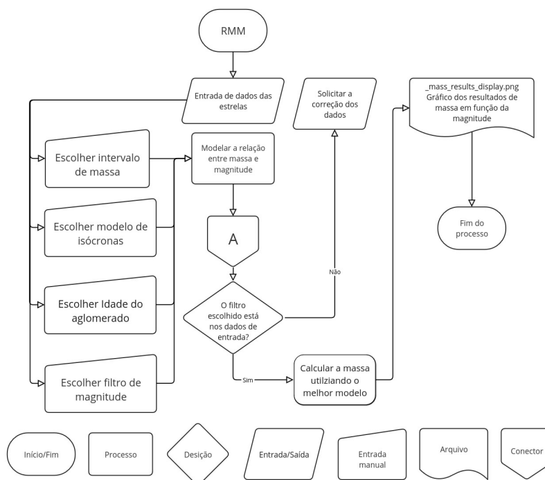
Figura 6 – Fluxograma do processo de relação massa-magnitude (RMM) para estimativa de massa estelar.
