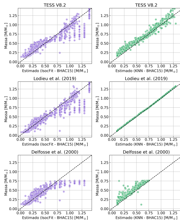
Figura 18 – Comparação entre estimativas de massa utilizando os métodos de ajuste de isócronas e relação massa-magnitude (KNN), ambos com o modelo BHAC15. Cada linha representa um conjunto de dados diferente: Stassun et al. (2019), Lodieu et al. (2019), e Delfosse et al. (2000). A primeira coluna refere-se ao método de ajuste de isócronas, enquanto a segunda representa a relação massa-magnitude. A linha tracejada indica a linha de identidade, onde a estimativa e o valor de referência são iguais.
