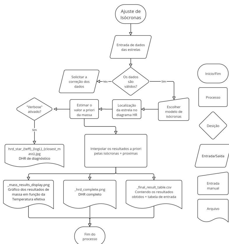
Figura 4 – Fluxograma do processo de ajuste de isócronas para estimativa de parâmetros estelares.
