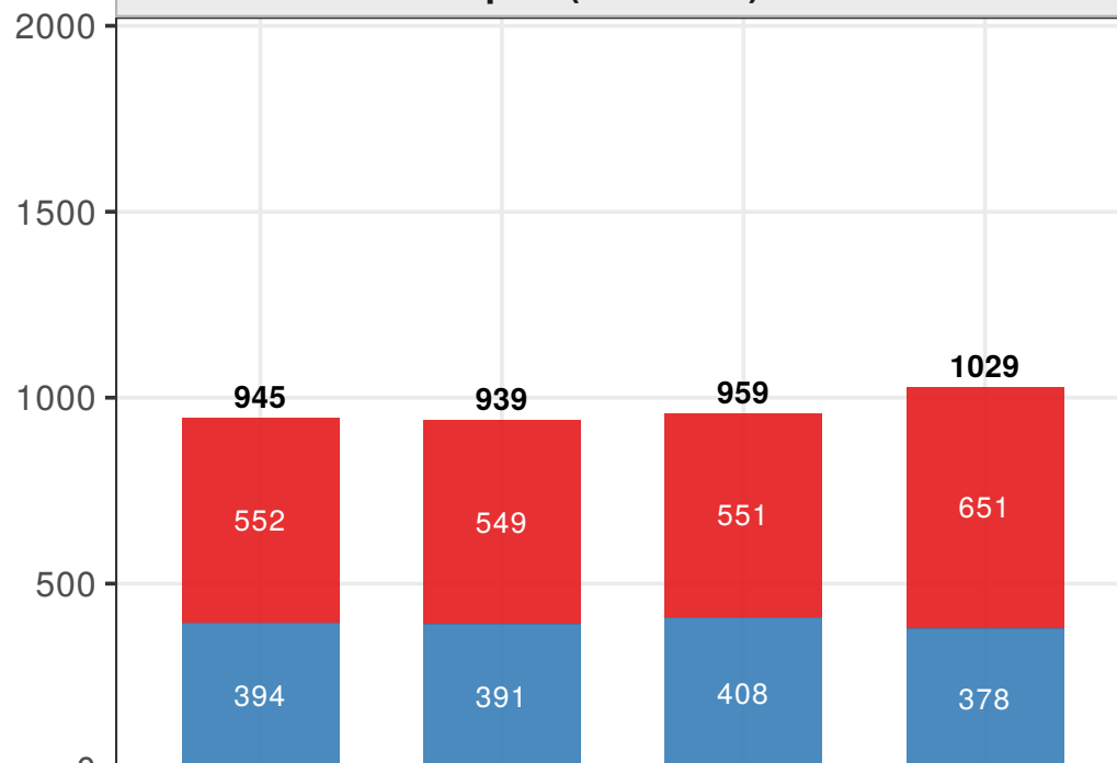
poti (RTX 4070)
