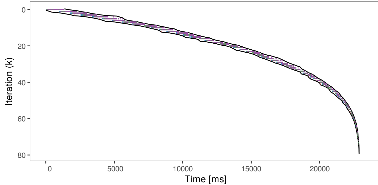
parsec:lfq
