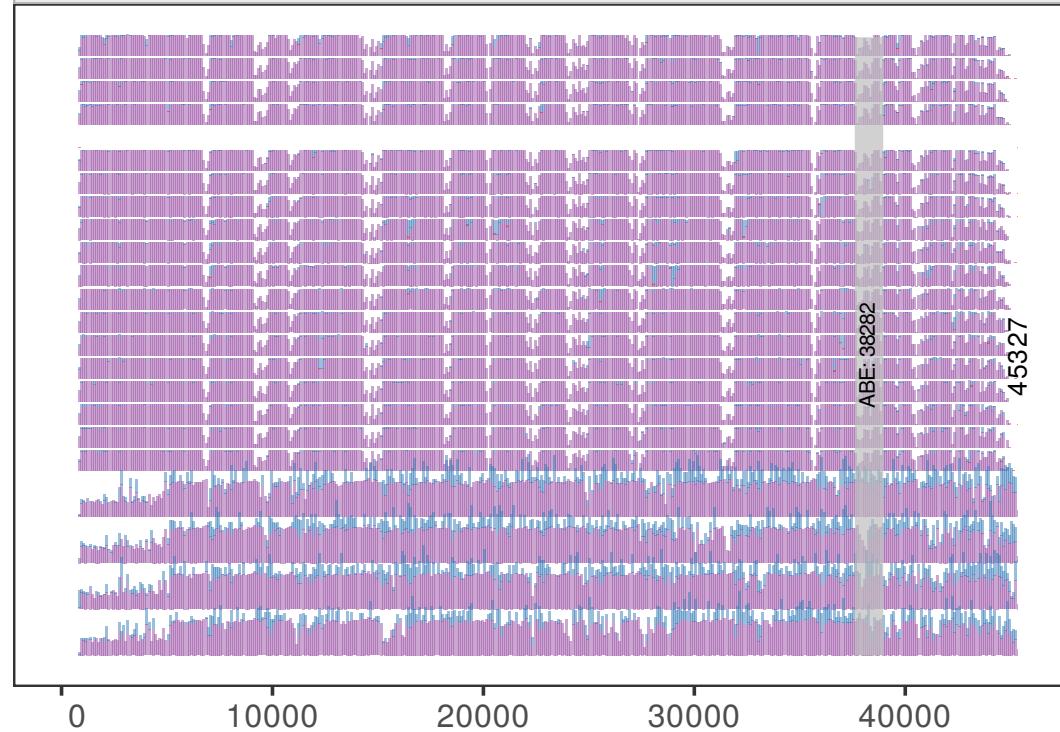
parsec:lfq
