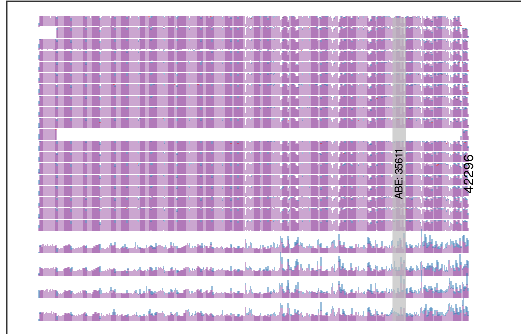
parsec:lfq
