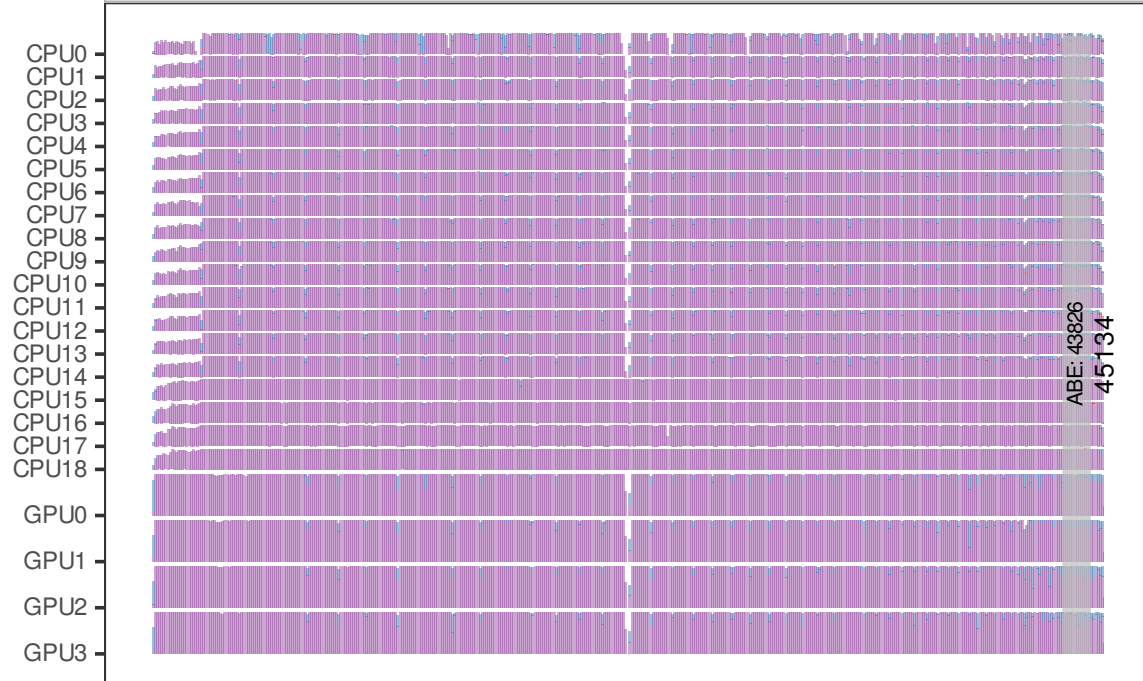
starpu:dmdas
