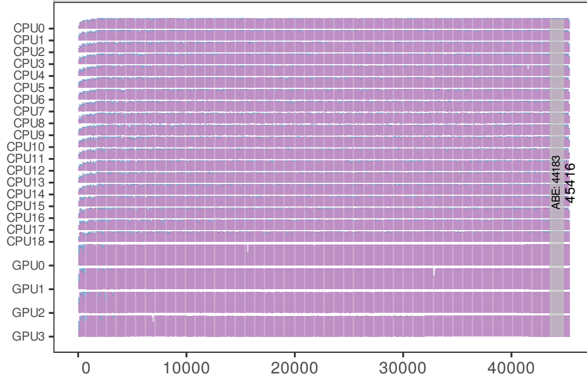
starpu:dmdas
