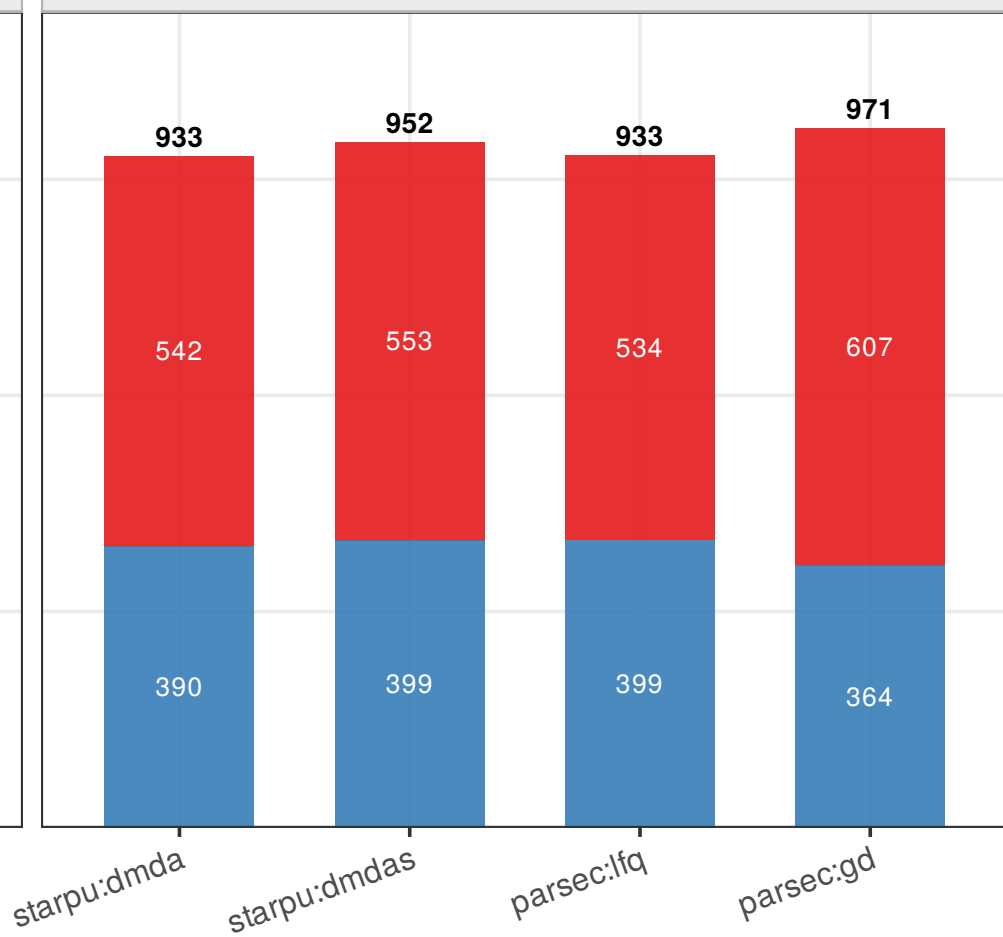
potrf
