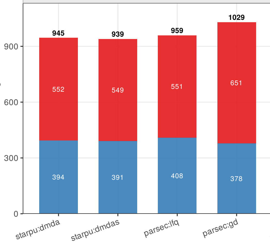
getrf_nopiv
