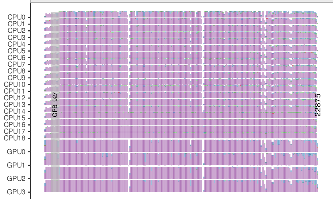
starpu:dmda
