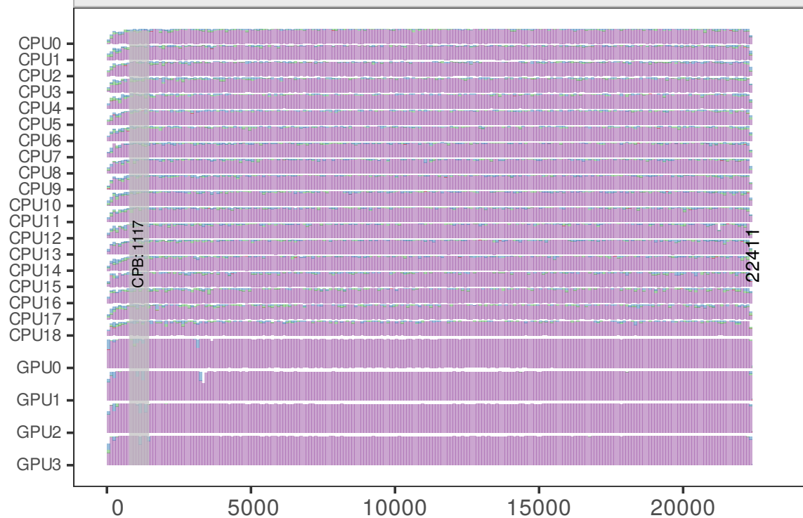
starpu:dmdas
