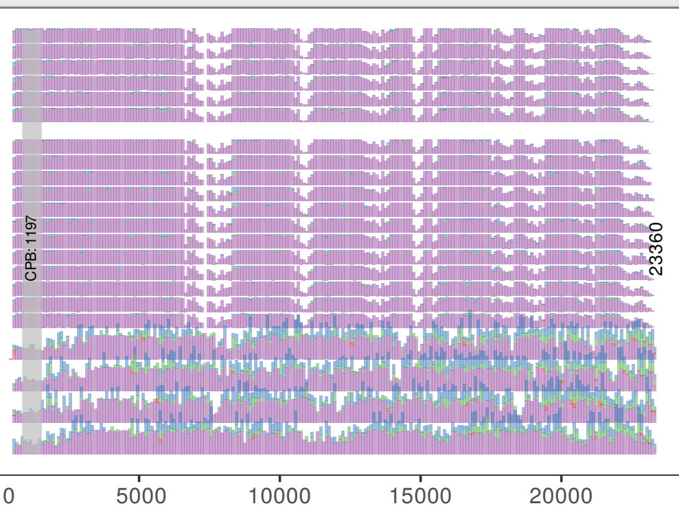
parsec:lfq
