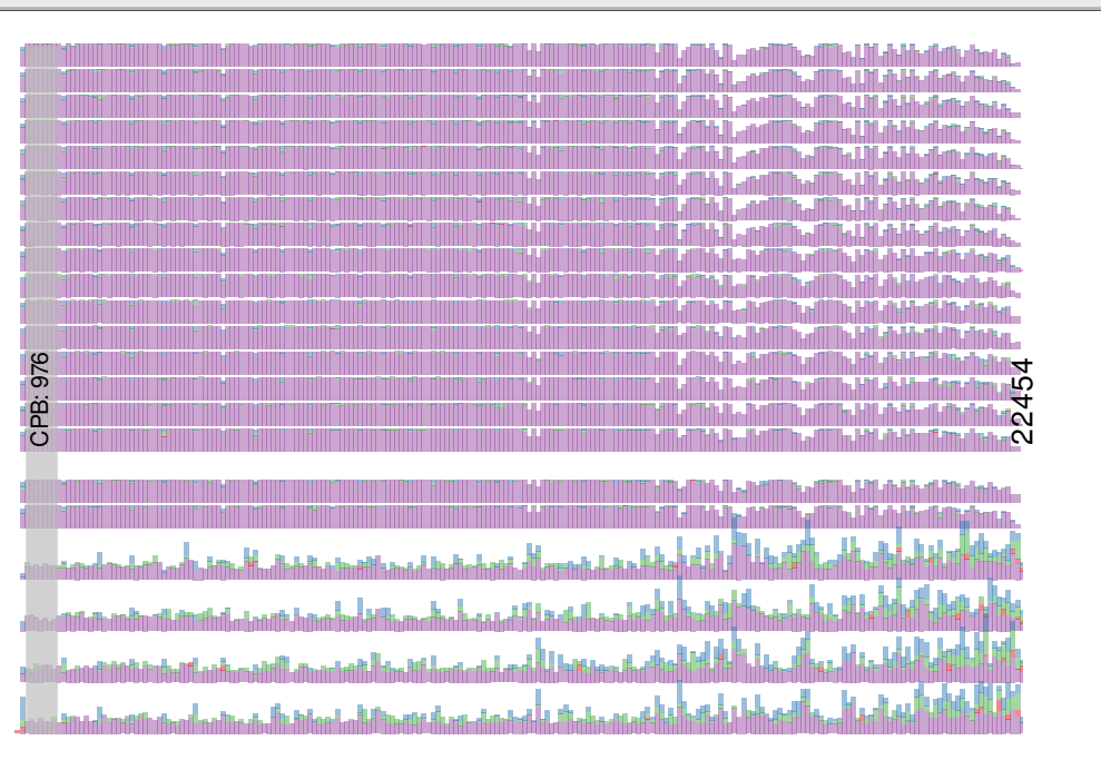
parsec:gd
