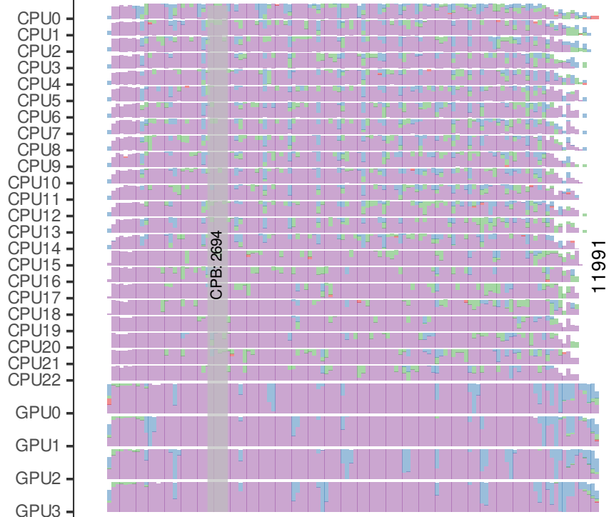
starpu:dmdas
