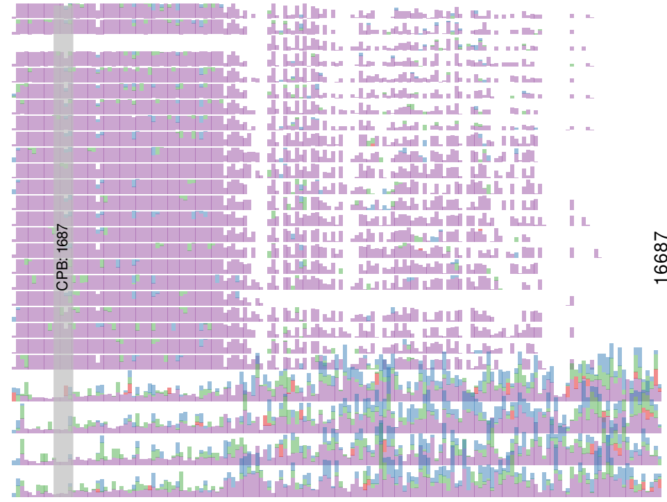
parsec:lfq
