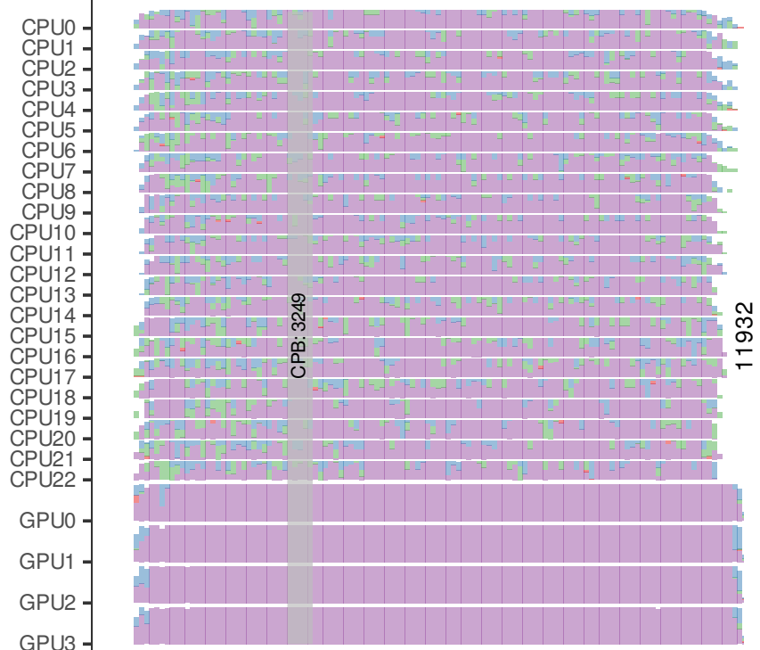
starpu:dmdas
