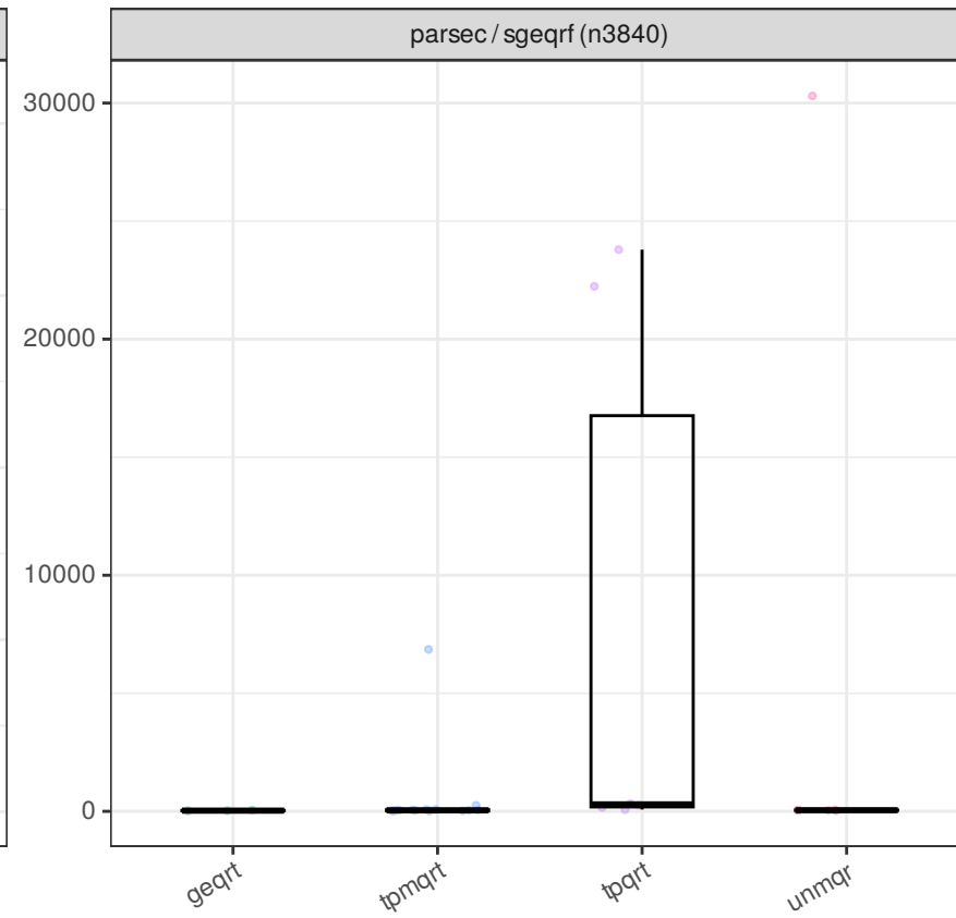
Tempo de escalonamento por tarefa (atraso entre ficar pronta e iniciar)
