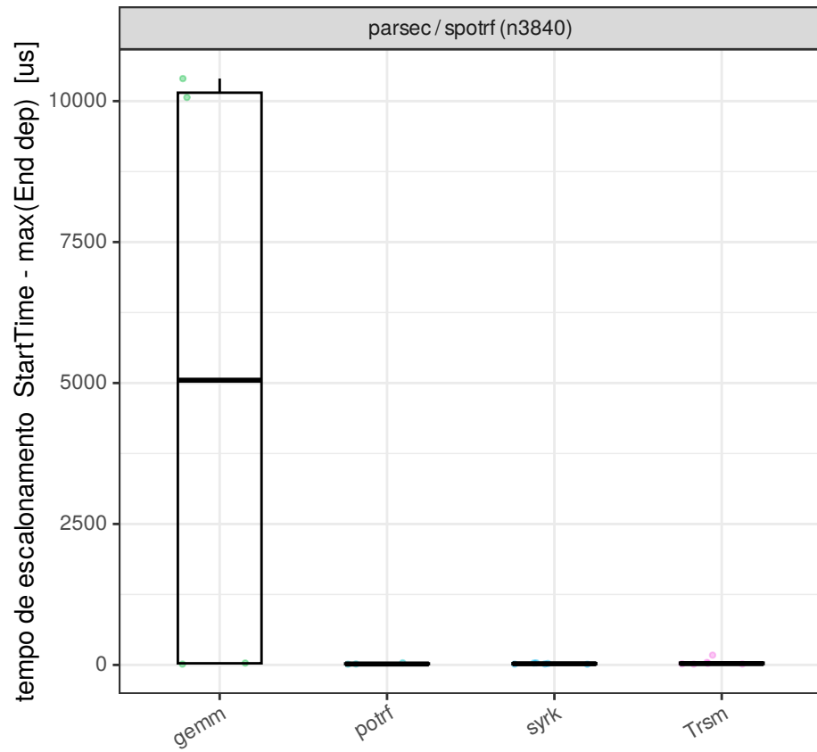
Tempo de escalonamento por tarefa (atraso entre ficar pronta e iniciar)
