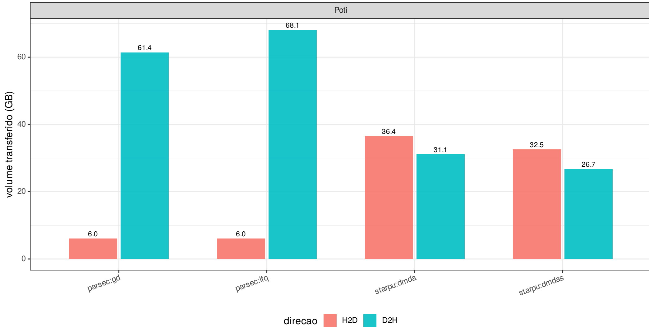
Trafergo PCIe H2D/D2H por runtime:scheduler
