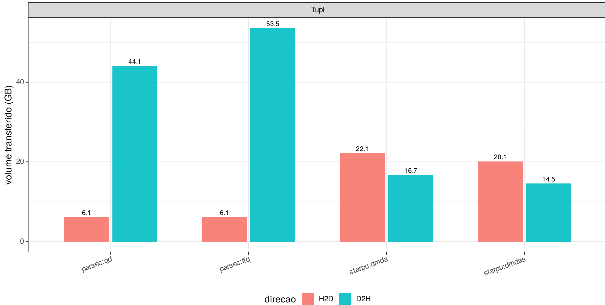
Trafego PCIe H2D/D2H por runtime:scheduler
