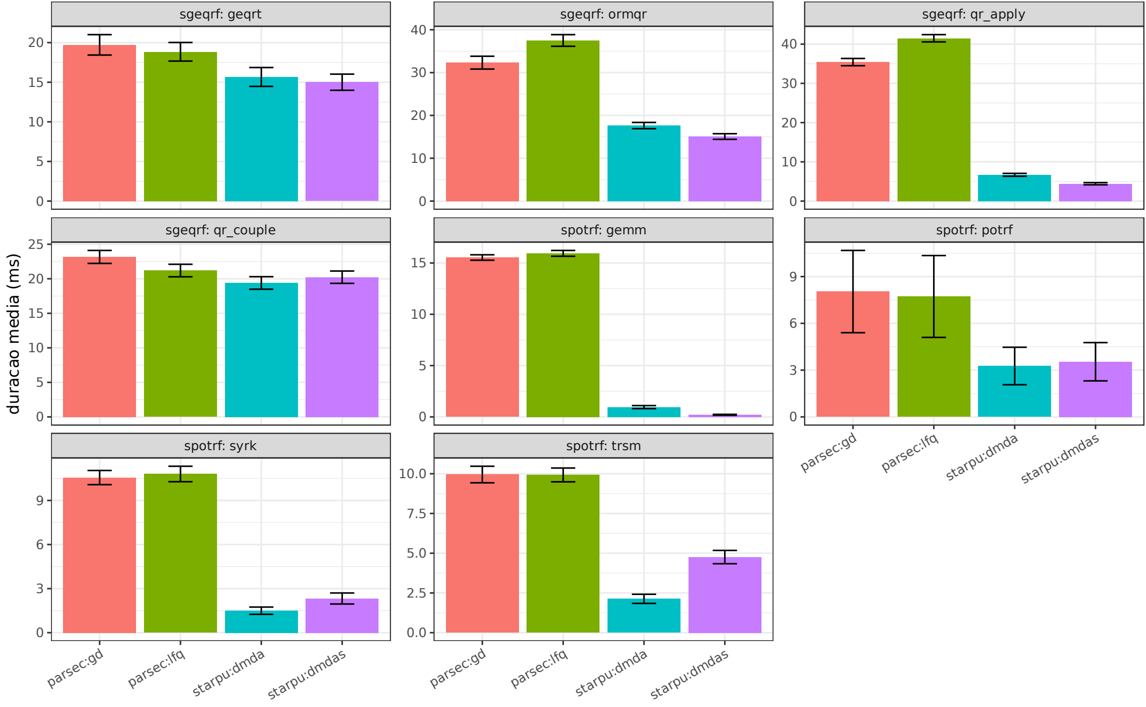
Tempo medio por tipo de tarefa (kernel) x runtime:scheduler data/manual_traces_20260621_172820/runs
