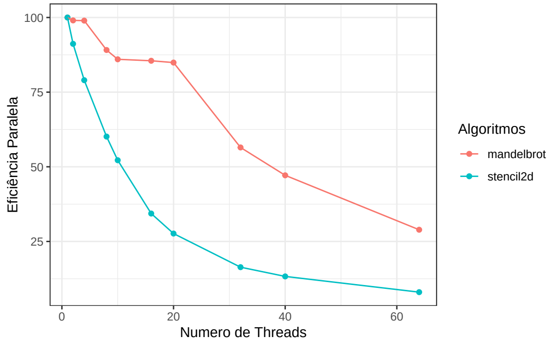
Eficiência Paralela pelo número de threads
